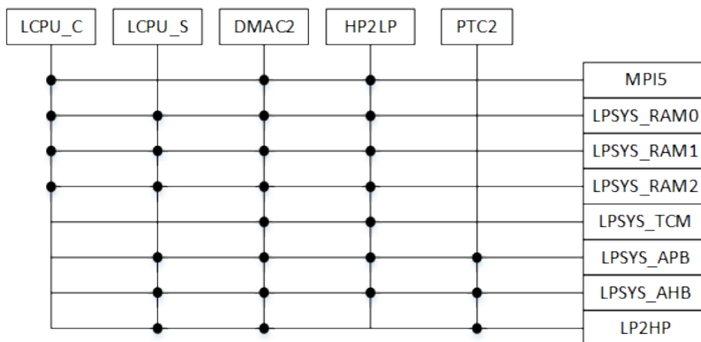
图 1-3: 低功耗处理器（小核）系统总线架构
