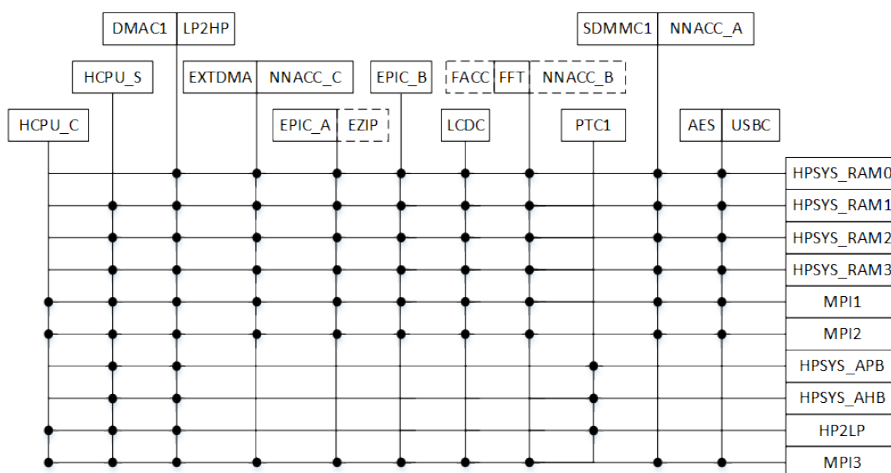
图 1-1: 性能处理器（大核）系统总线架构 HCPU
