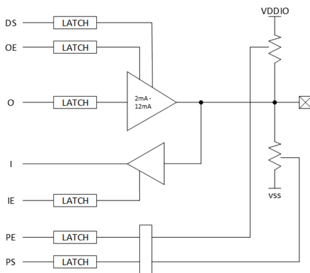
图 5-1: IO 结构
