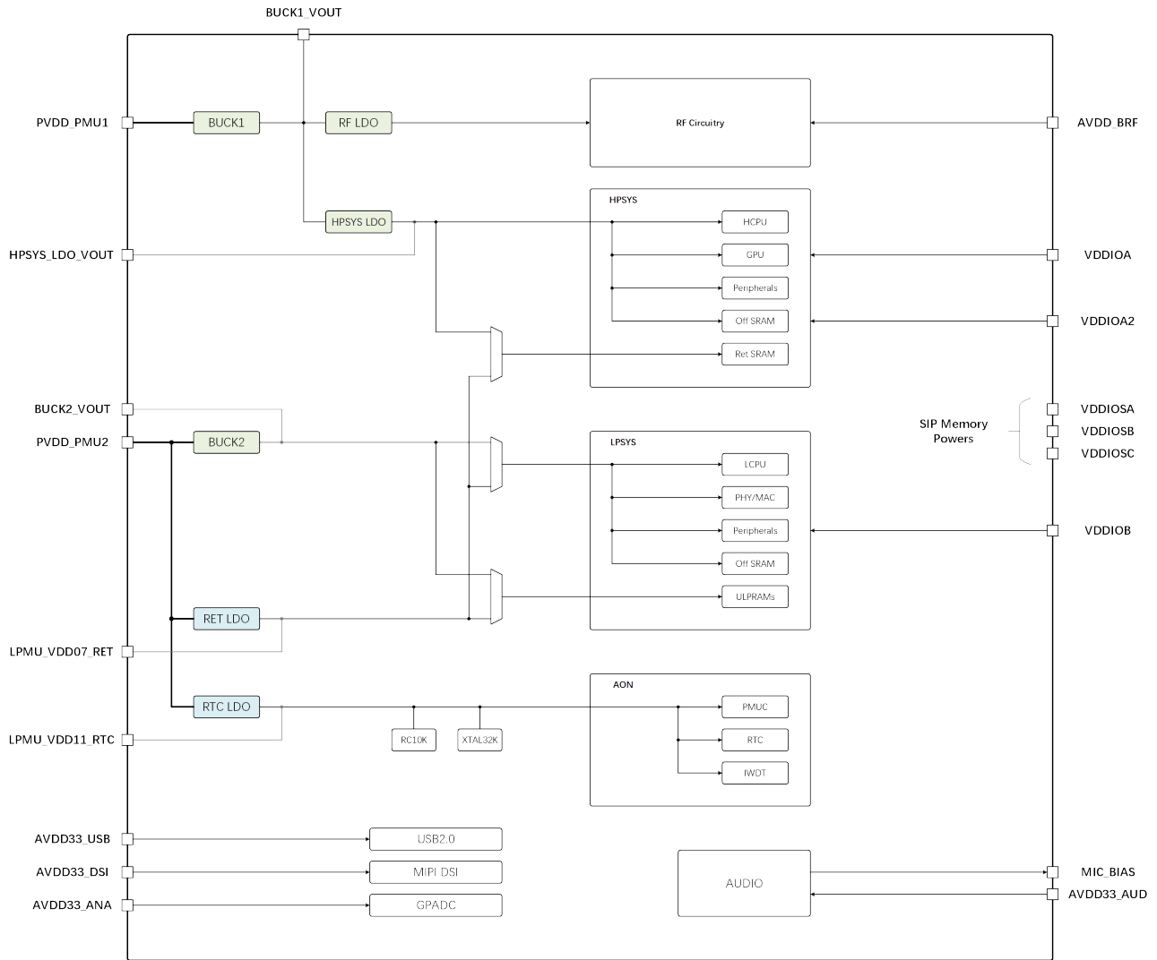
图 3-1: 电源管理架构
