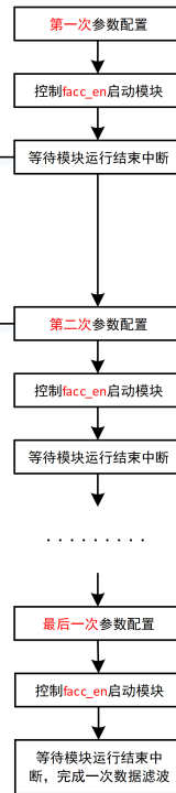
图 12-1: 非缓存模式下的配置流程图
