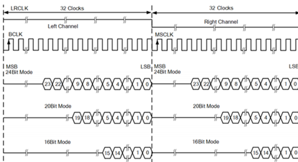
图 10-6: I2S 右对齐
