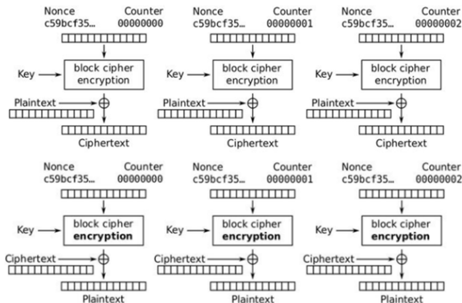
图 12-2: CTR 模式解密
