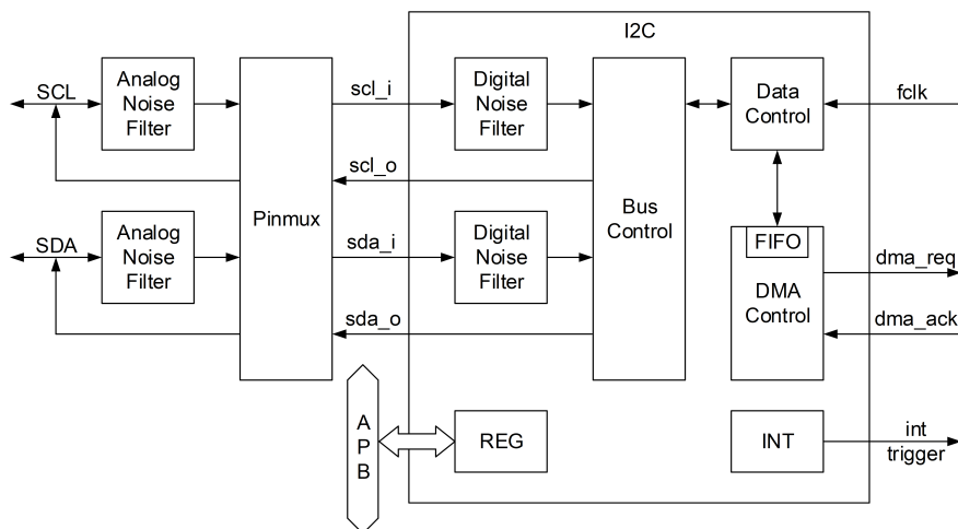
图 6-1: I2C 结构图
