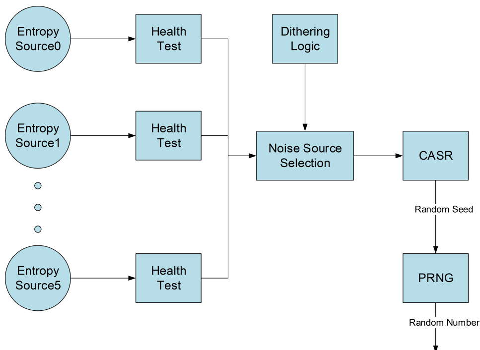
图 12-4: TRNG 结构图
