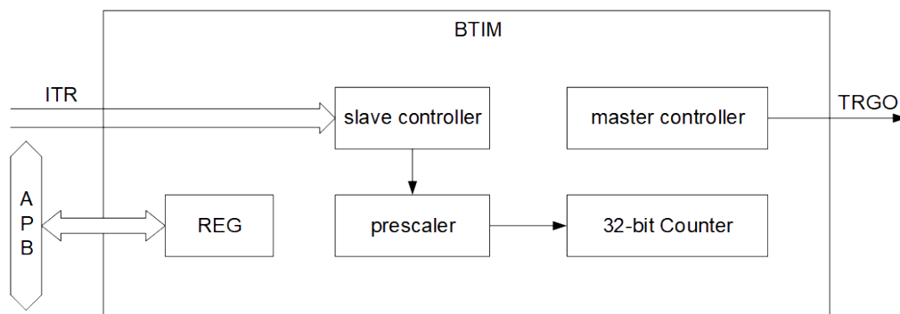
图 8-7: BTIM 结构图
