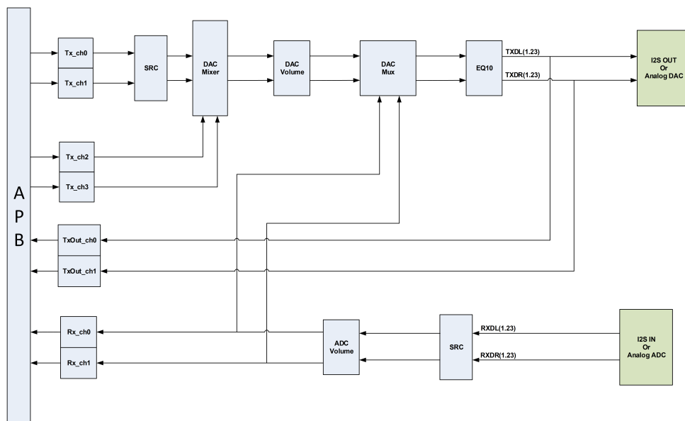
图 10-7: Audprc 结构图
