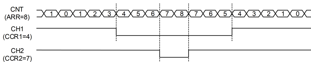
图 8-10: 中心对齐计数模式下的 PWM 输出
