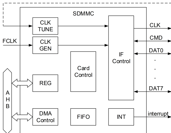
图 13-1: SDMMC 结构图
