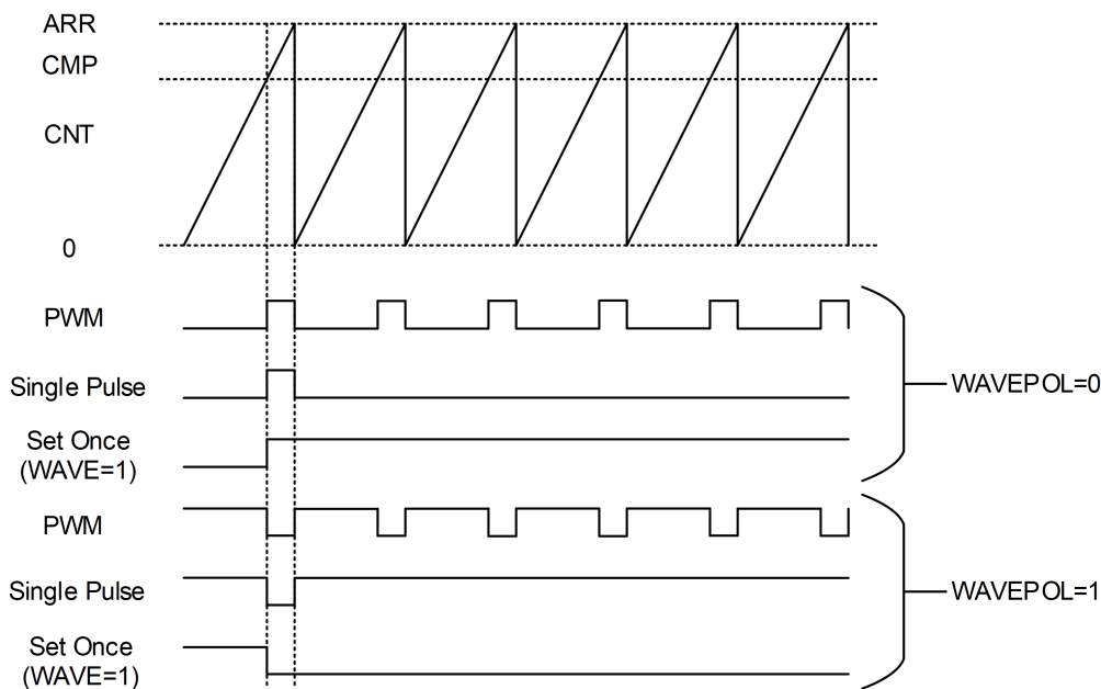
图 8-14: PWM 输出
