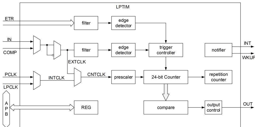
图 8-13: LPTIM 结构图
