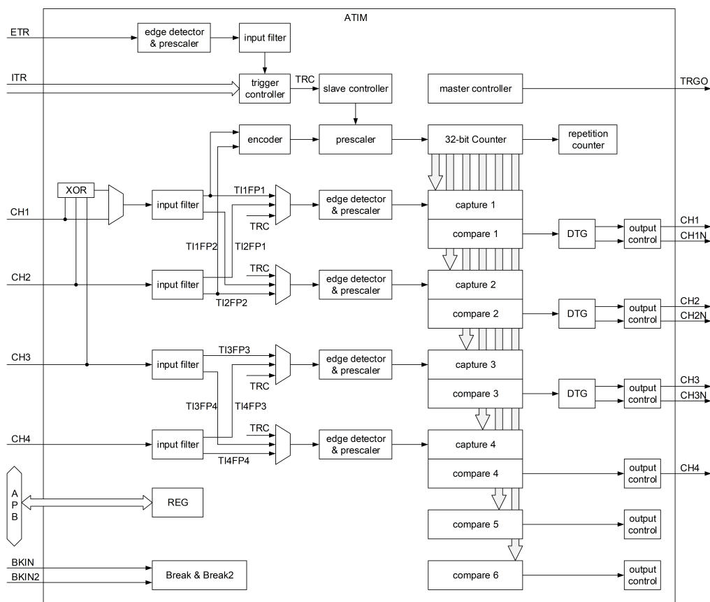
图 8-1: ATIM 结构图
