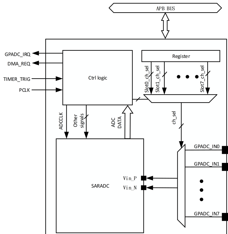
图 7-1: GPADC 框图
