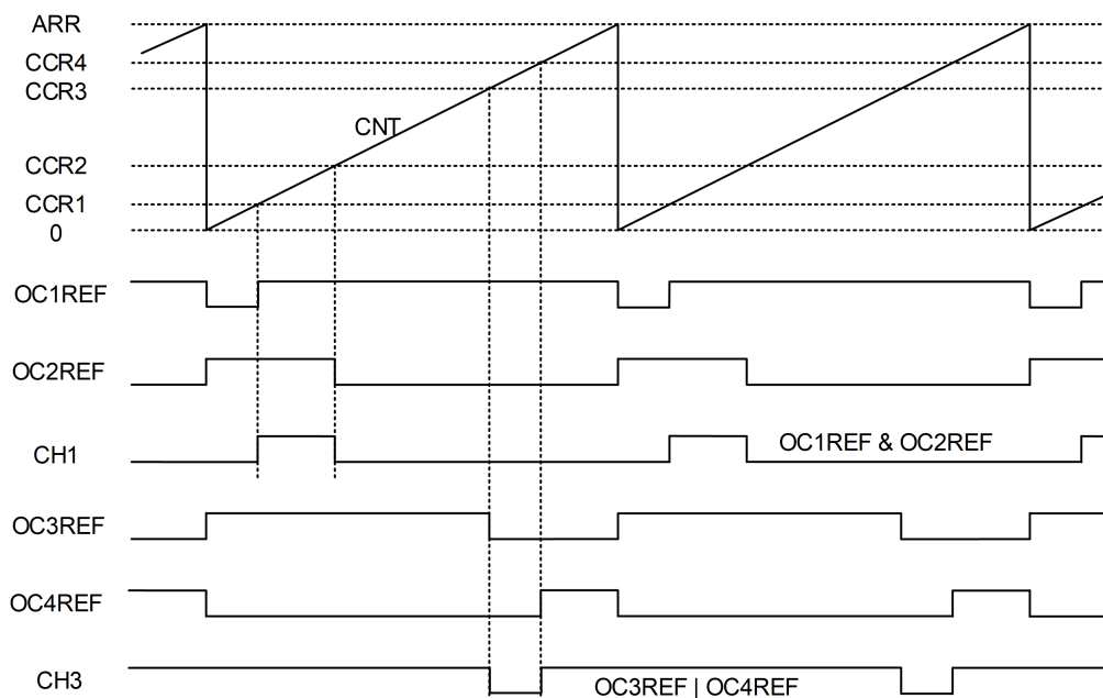
图 8-5: 组合 PWM 输出
