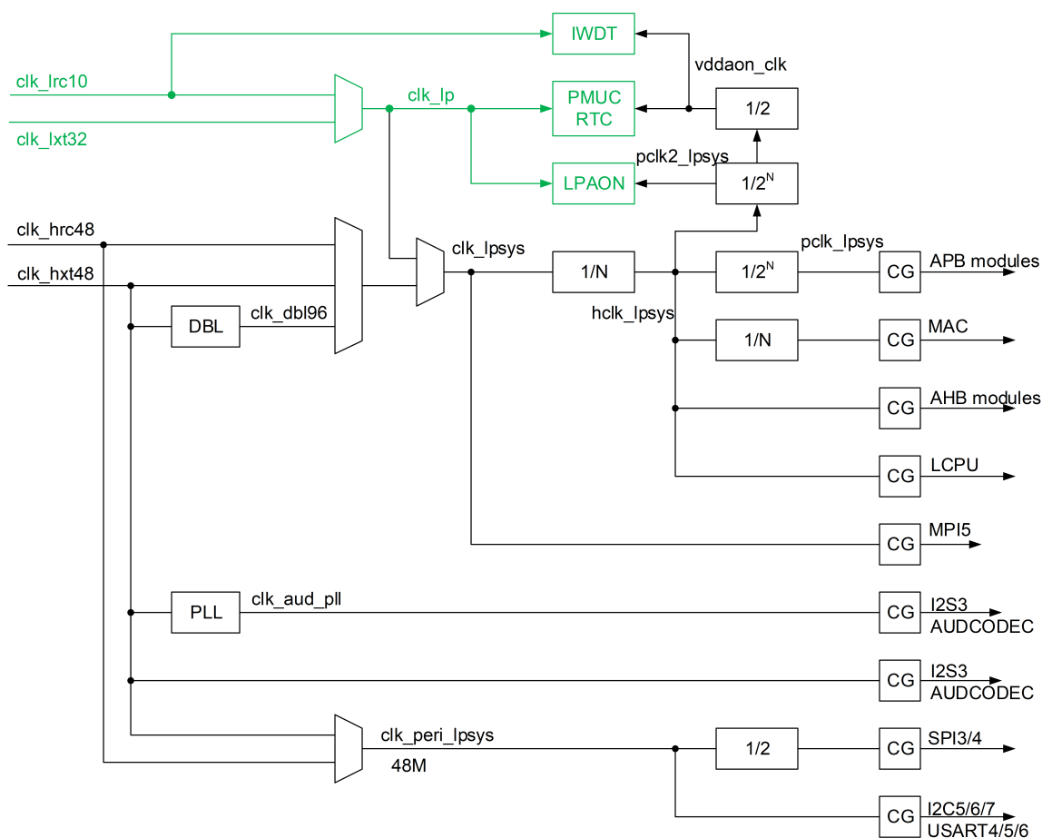
图 2-2: LPSYS 时钟结构
