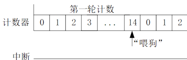
图 8-17: 模式 1 “喂狗”行为对计数器的影响（假定超时值为 20）
