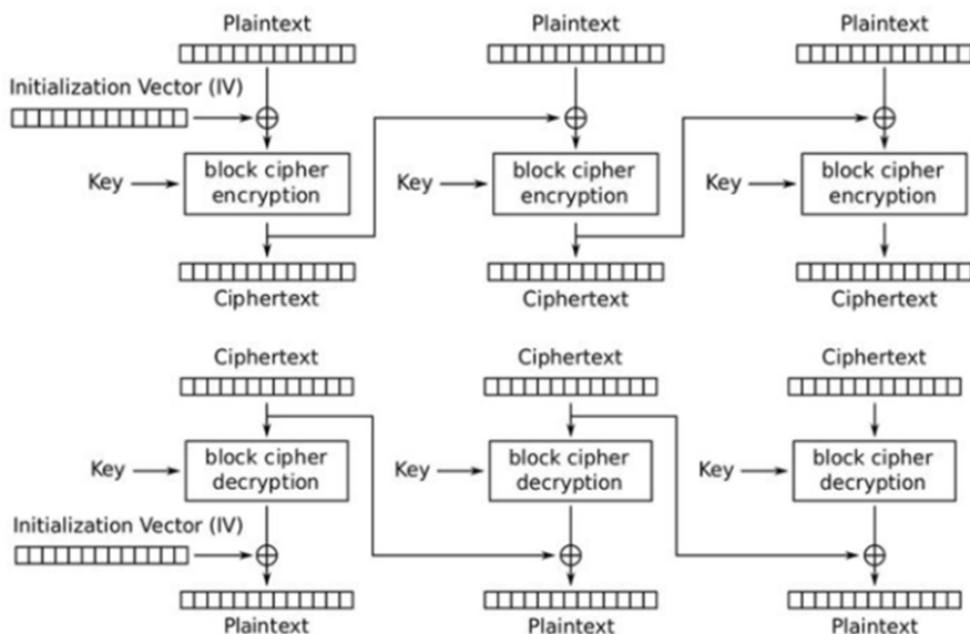
图 12-3: CBC 模式解密
