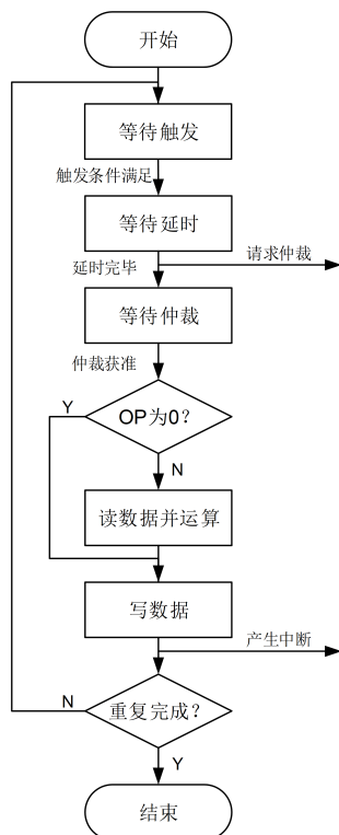
图 6-10: PTC 通道执行流程图
