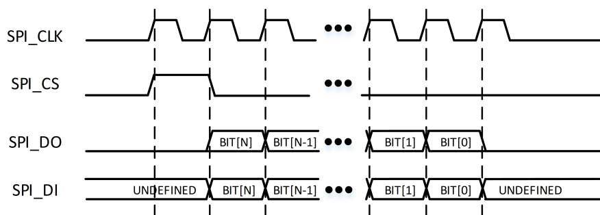
图 6-6: TI-SSP 协议通信时序
