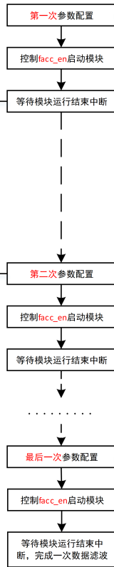
图 11-2: 缓存模式下的配置流程图
