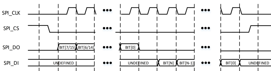
图 6-8: Microwire 协议单次通信时序
