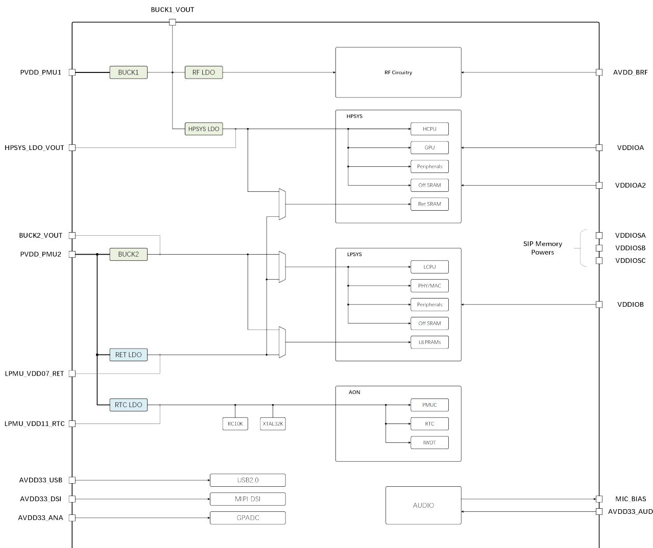
图 1-4: 电源管理架构
