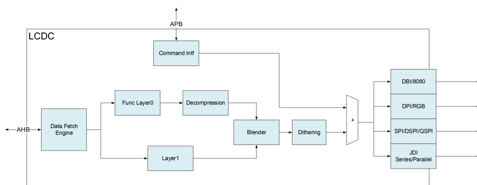
图 9-1: LCDC 架构图
