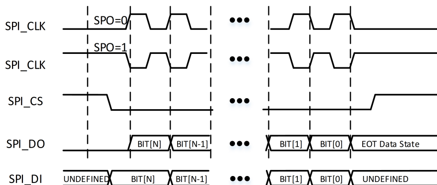
图 6-5: SPI 协议连续传输时序
