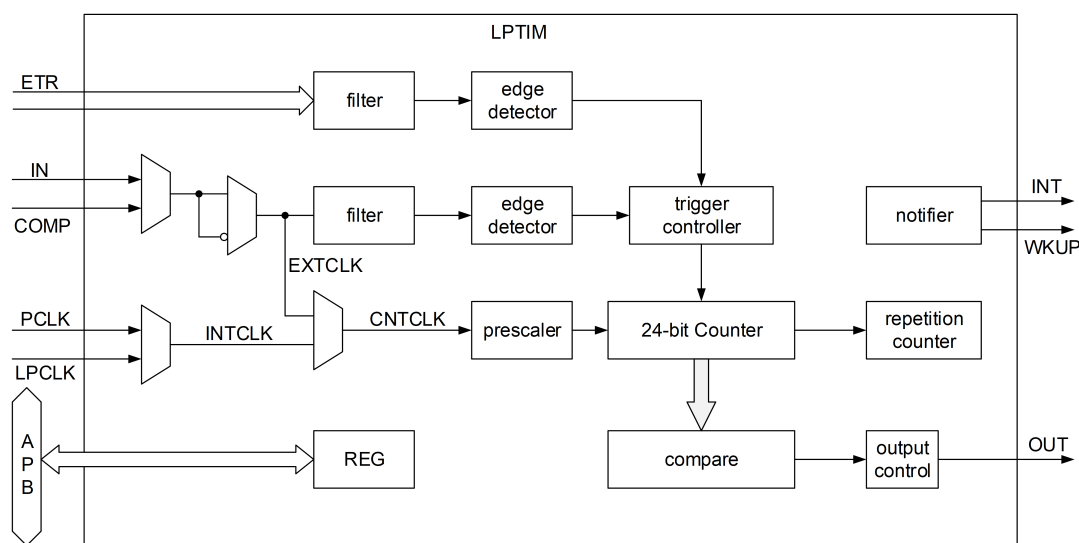
图 9-8: GPTIM 结构图
