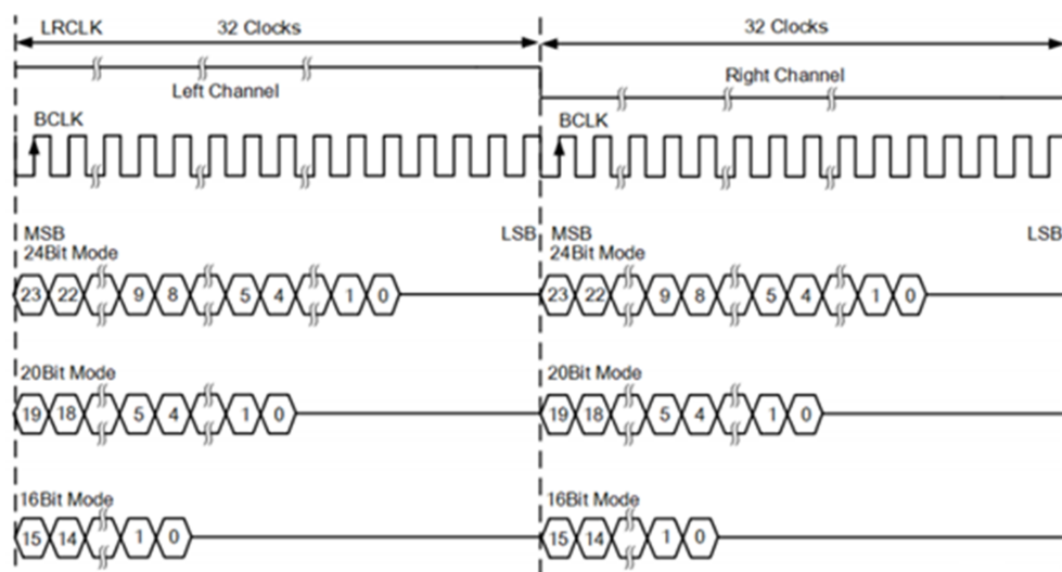
图 11-5: I2S 左对齐
