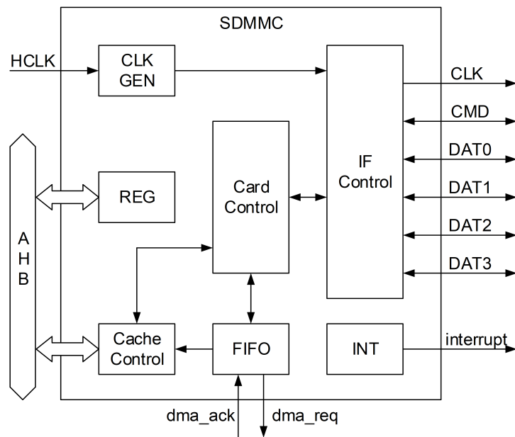
图 14-3: SDMMC 结构图
