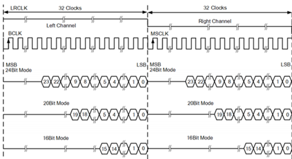
图 11-6: I2S 右对齐
