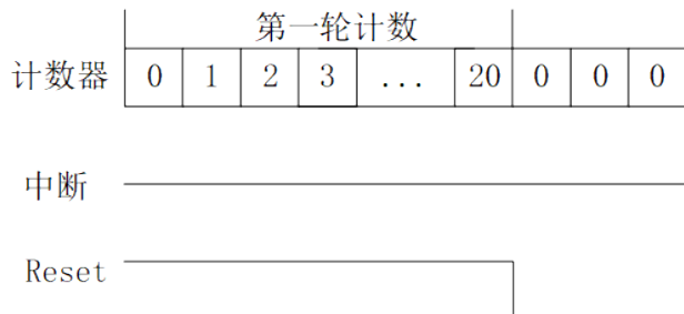
图 9-9: 模式 1 的中断以及 reset 信号产生与计数器的关系（假定超时值为 20，reset 低有效）
