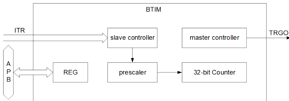
图 9-1: BTIM 结构图
