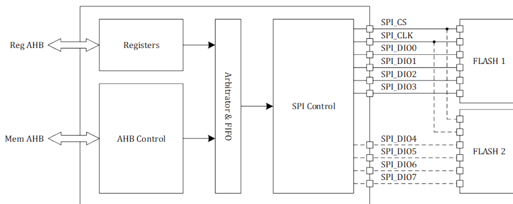
图 14-3: QSPI 控制器框图
