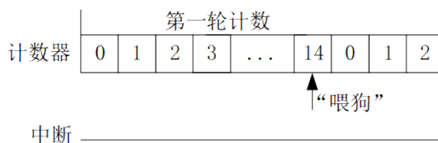
图 9-11: 模式 1 “喂狗”行为对计数器的影响（假定超时值为 20）
