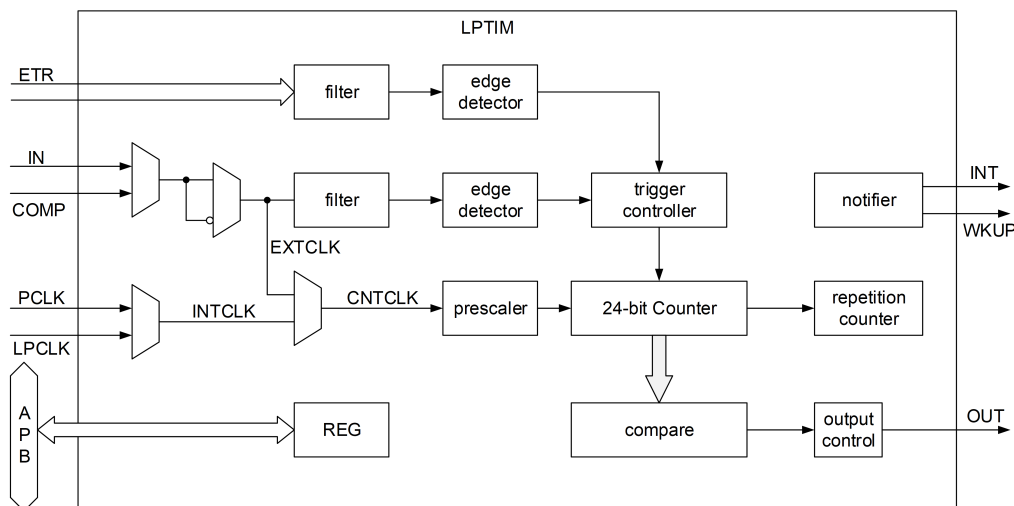
图 9-7: LPTIM 结构图
