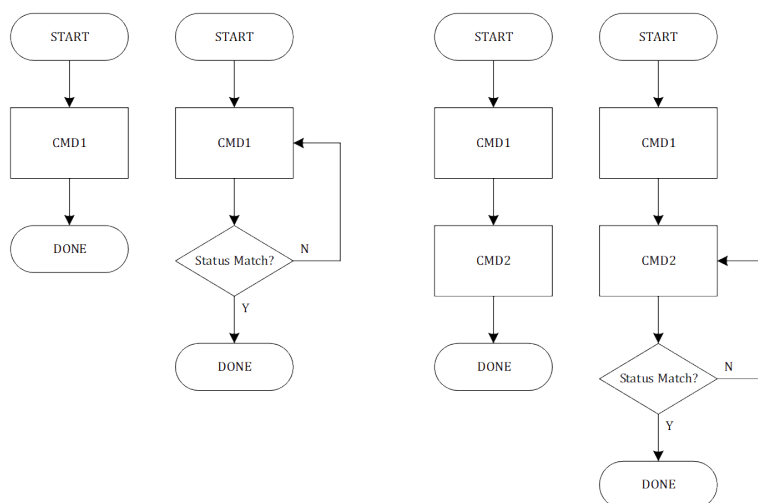
图 14-4: 寄存器模式单个和多个命令时序的序列
