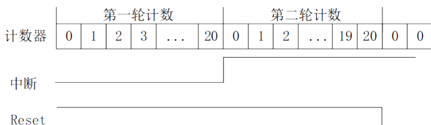
图 9-10: 模式 2 的中断以及 reset 信号产生与计数器的关系（假定超时值为 20，reset 低有效）
