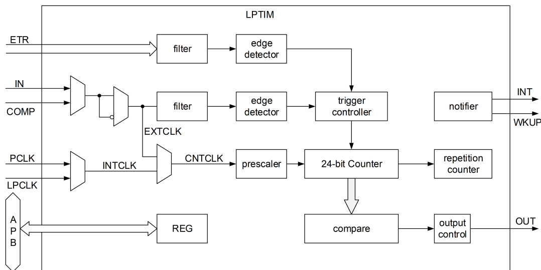
图 9-2: GPTIM 结构图
