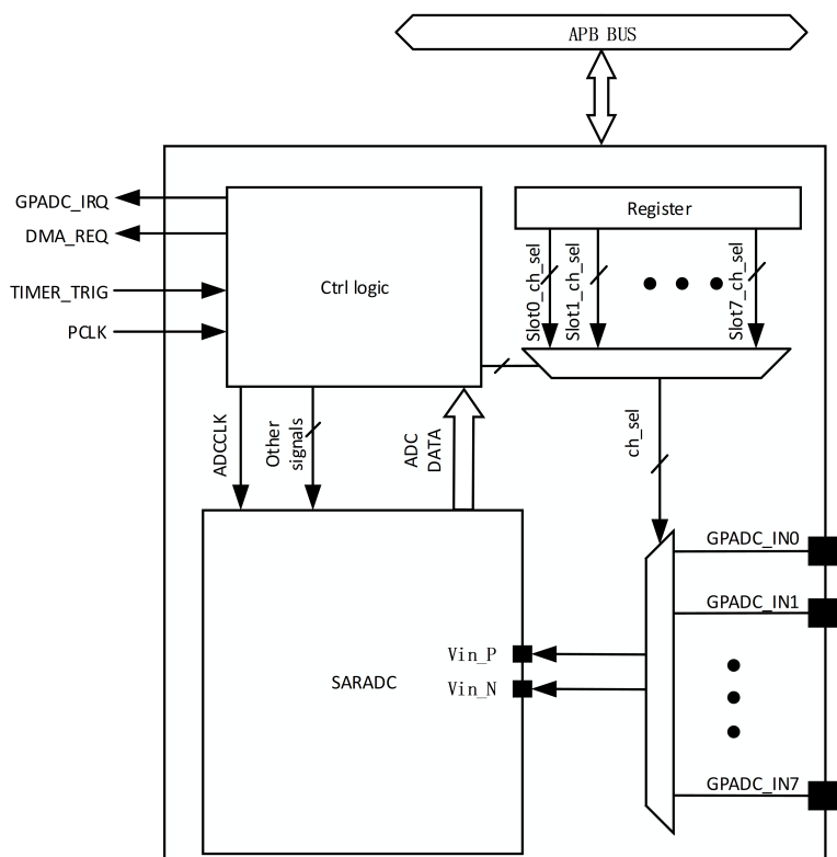
图 8-1: GPADC 框图
