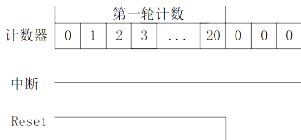
图 9-9: 模式 1 的中断以及 reset 信号产生与计数器的关系（假定超时值为 20，reset 低有效）
