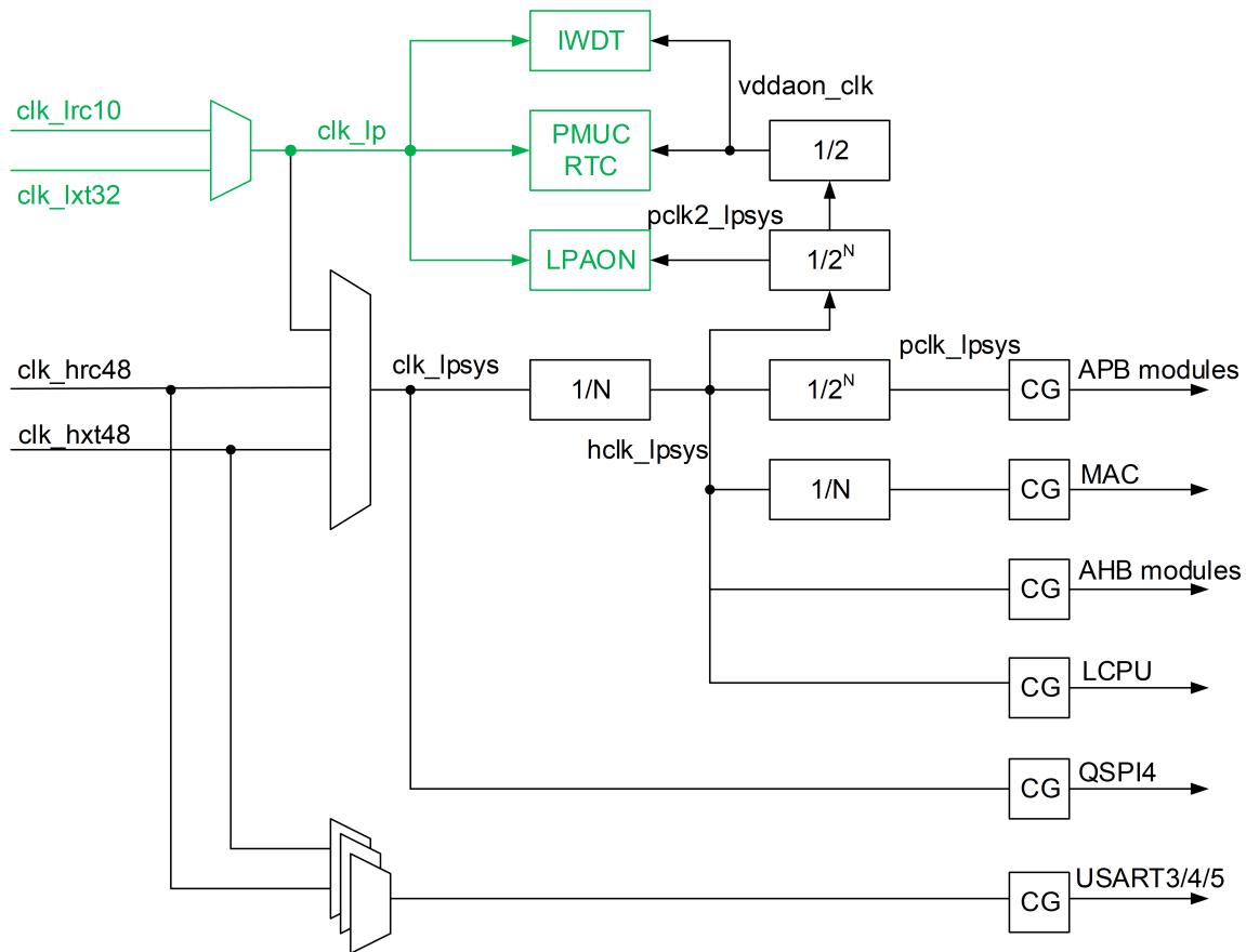
图 2-2: LPSYS 时钟结构
