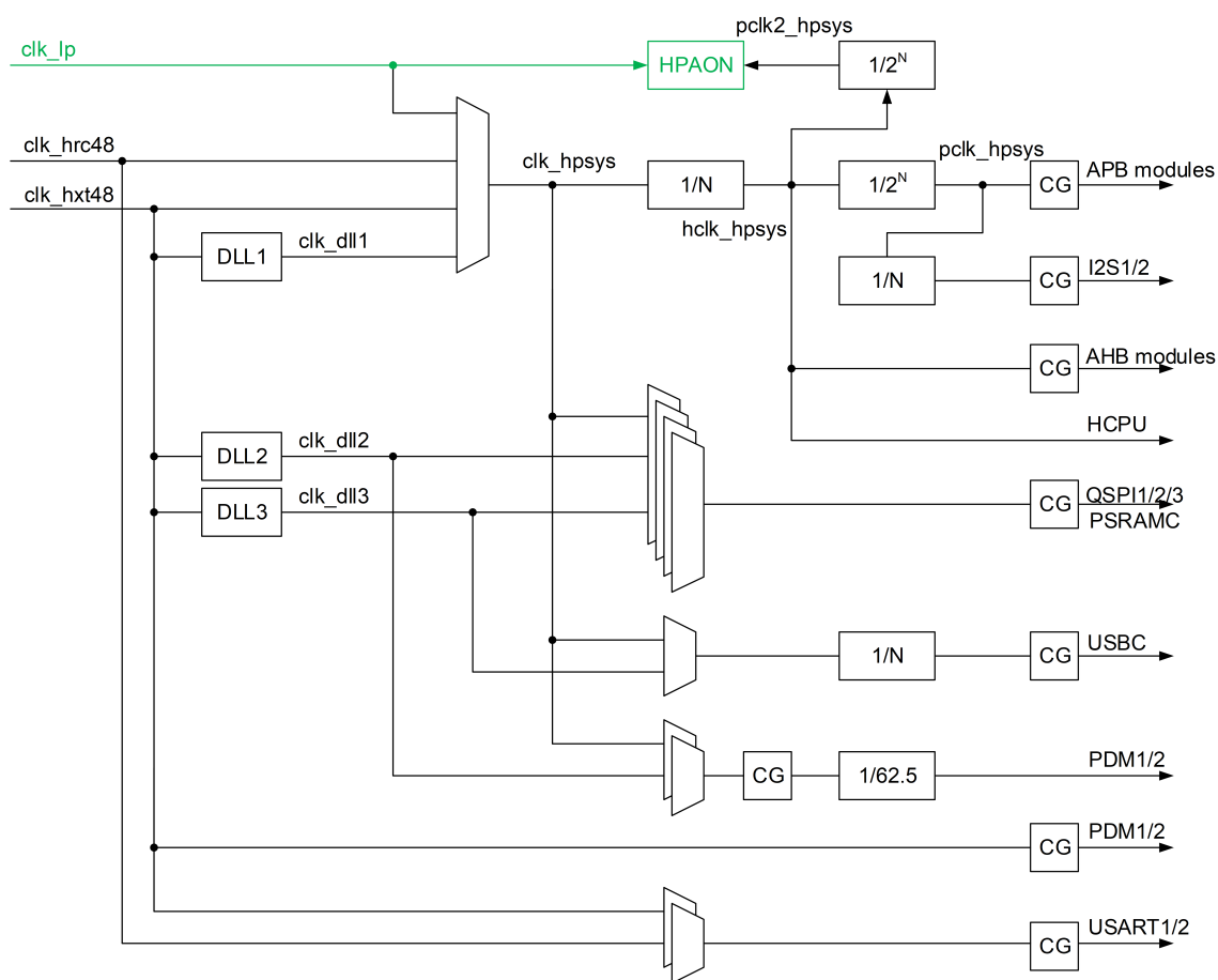
图 2-1: HPSYS 时钟结构
