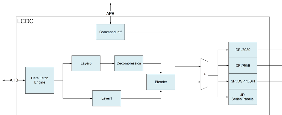
图 10-1: LCDC 架构图
