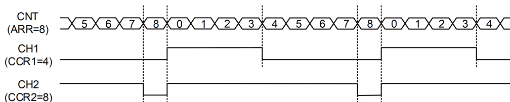
图 9-3: 递增计数模式下的 PWM 输出
