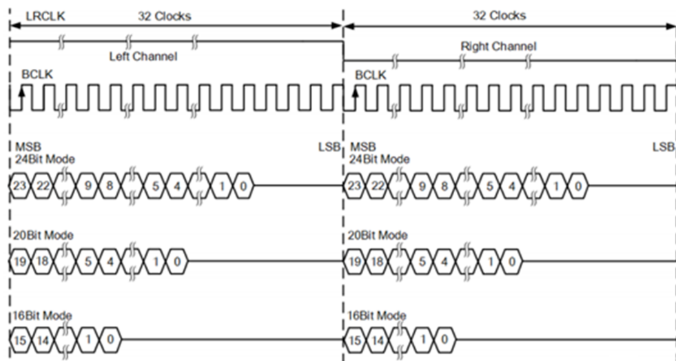
图 11-5: I2S 左对齐
