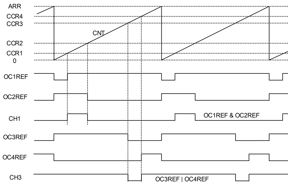
图 9-6: 组合 PWM 输出
