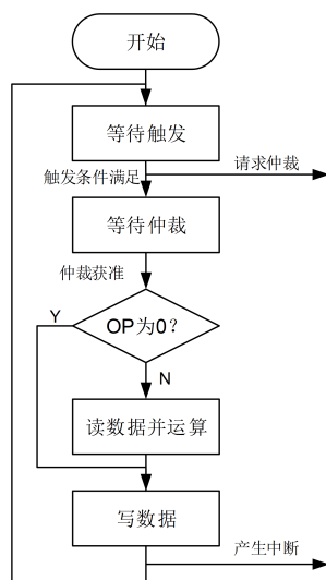
图 7-11: PTC 通道执行流程图
