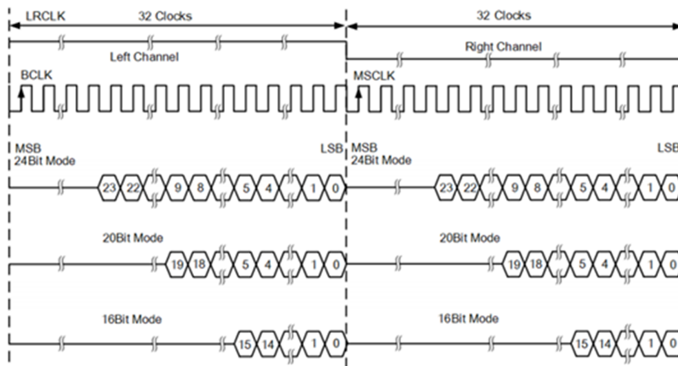
图 11-6: I2S 右对齐
