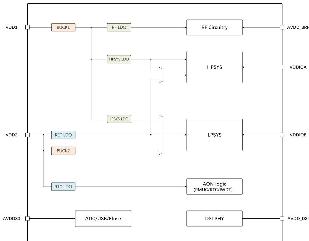
图 3-1: 电源管理架构
