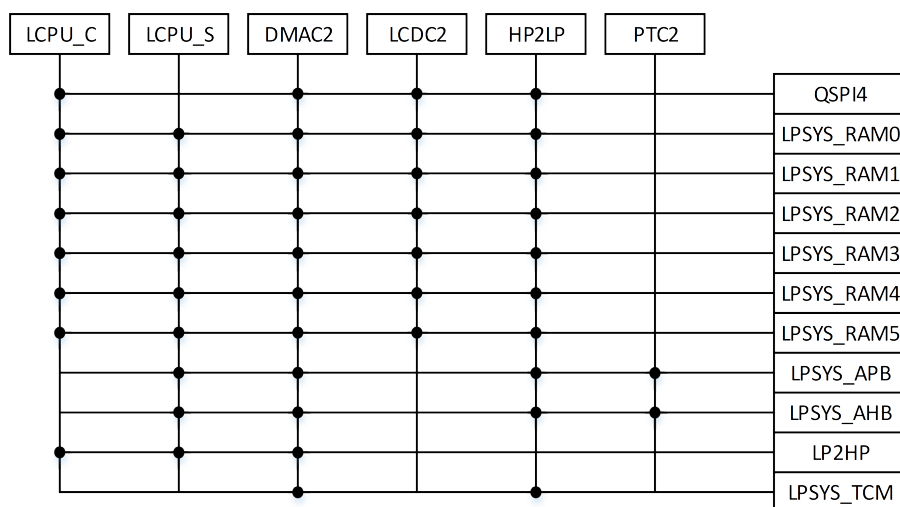
图 1-2: 低功耗处理器（小核）系统总线架构
