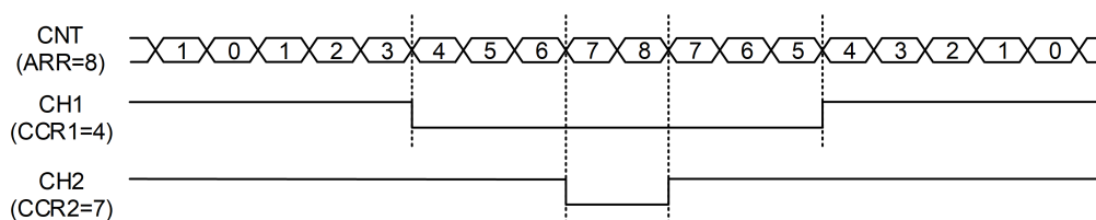
图 9-4: 中心对齐计数模式下的 PWM 输出
