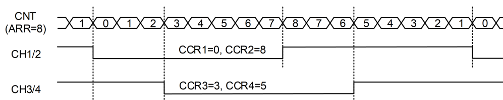
图 9-5: 不对称 PWM 输出
