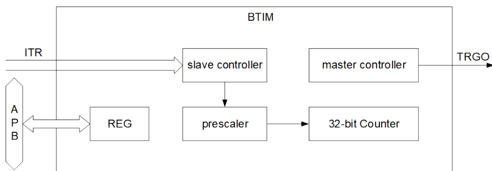
图 9-1: BTIM 结构图
