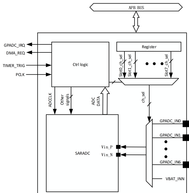
图 8-1: GPADC 框图
