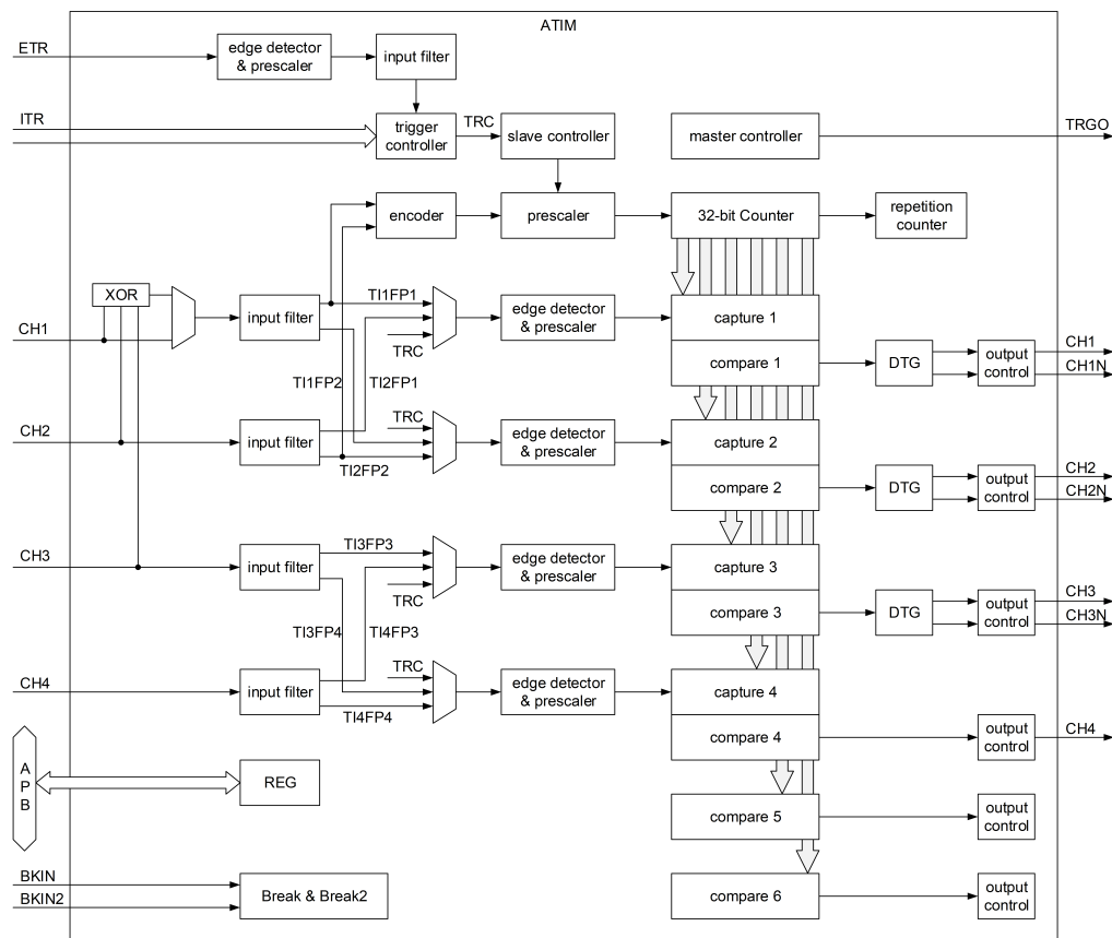
图 9-1: ATIM 结构图
