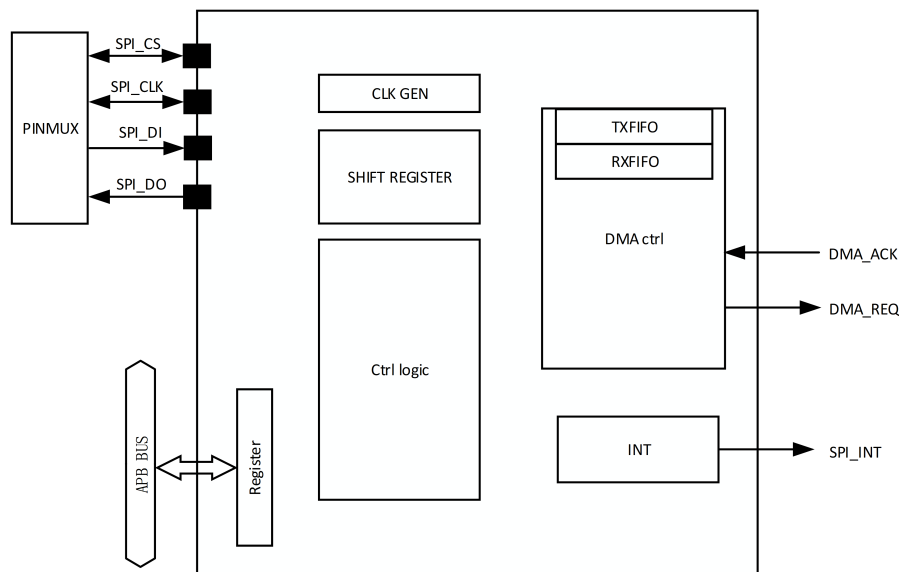
图 7-2: SPI 结构图
