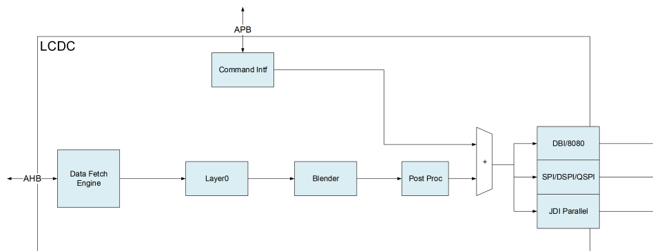
图 10-1: LCDC 架构图
