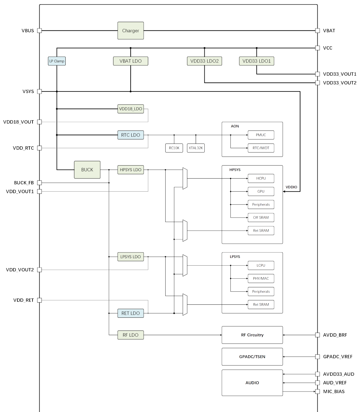
图 3-1: QFN 封装电源管理架构
