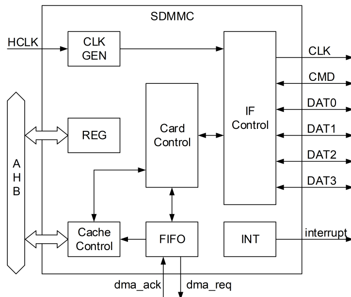
图 14-1: SDMMC 结构图
