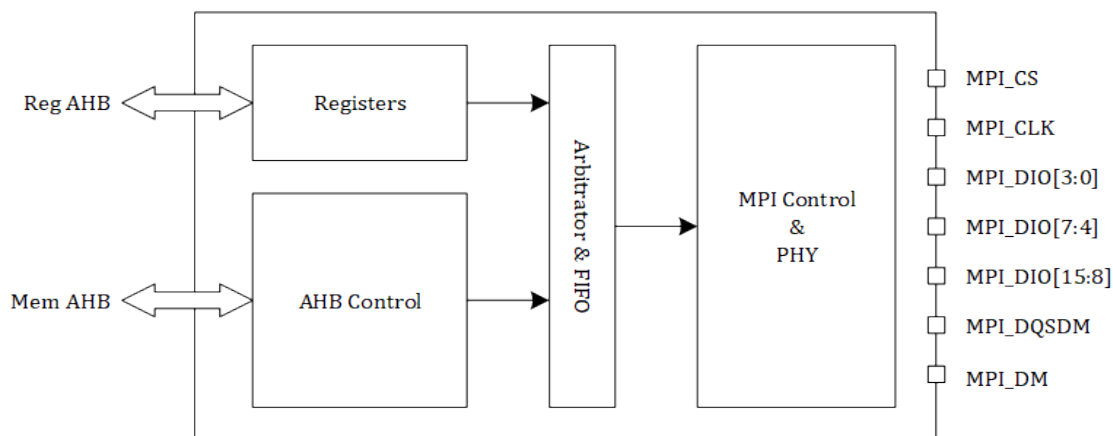
图 14-2: MPI 控制器框图
