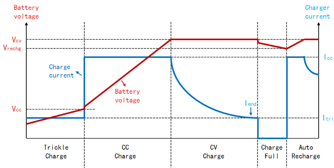
图 3-2: 充电曲线
