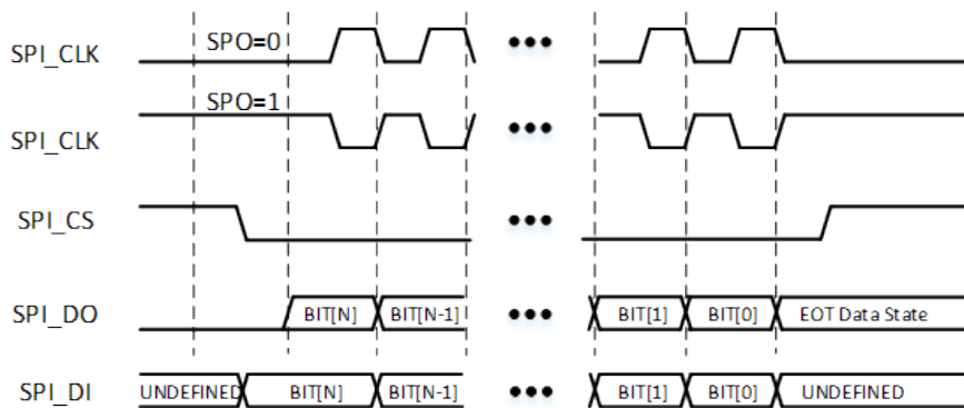
图 3-6: SPO=0 时的 SPI 时序
