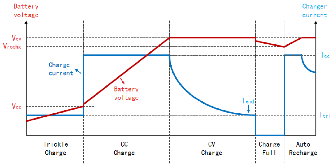
图 1-4: 充电曲线
