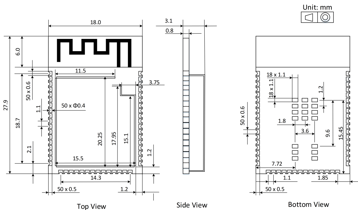
图 8-1: SF32LB52-MOD-1 模组尺寸图
