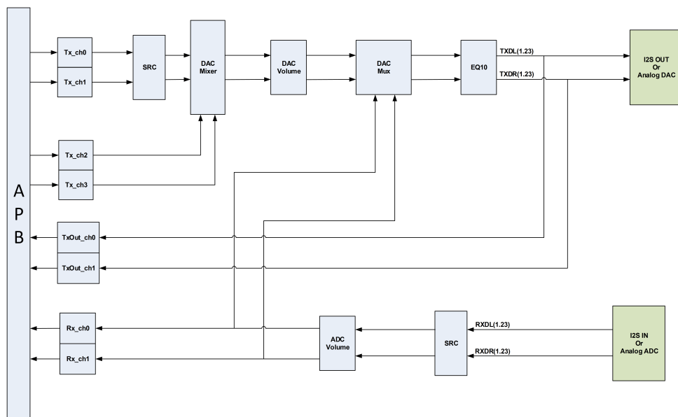
图 11-7: Audprc 结构图
