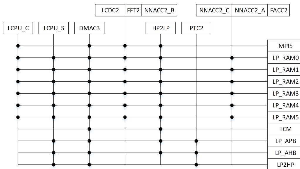
图 1-3: 低功耗处理器（小核）系统总线架构
