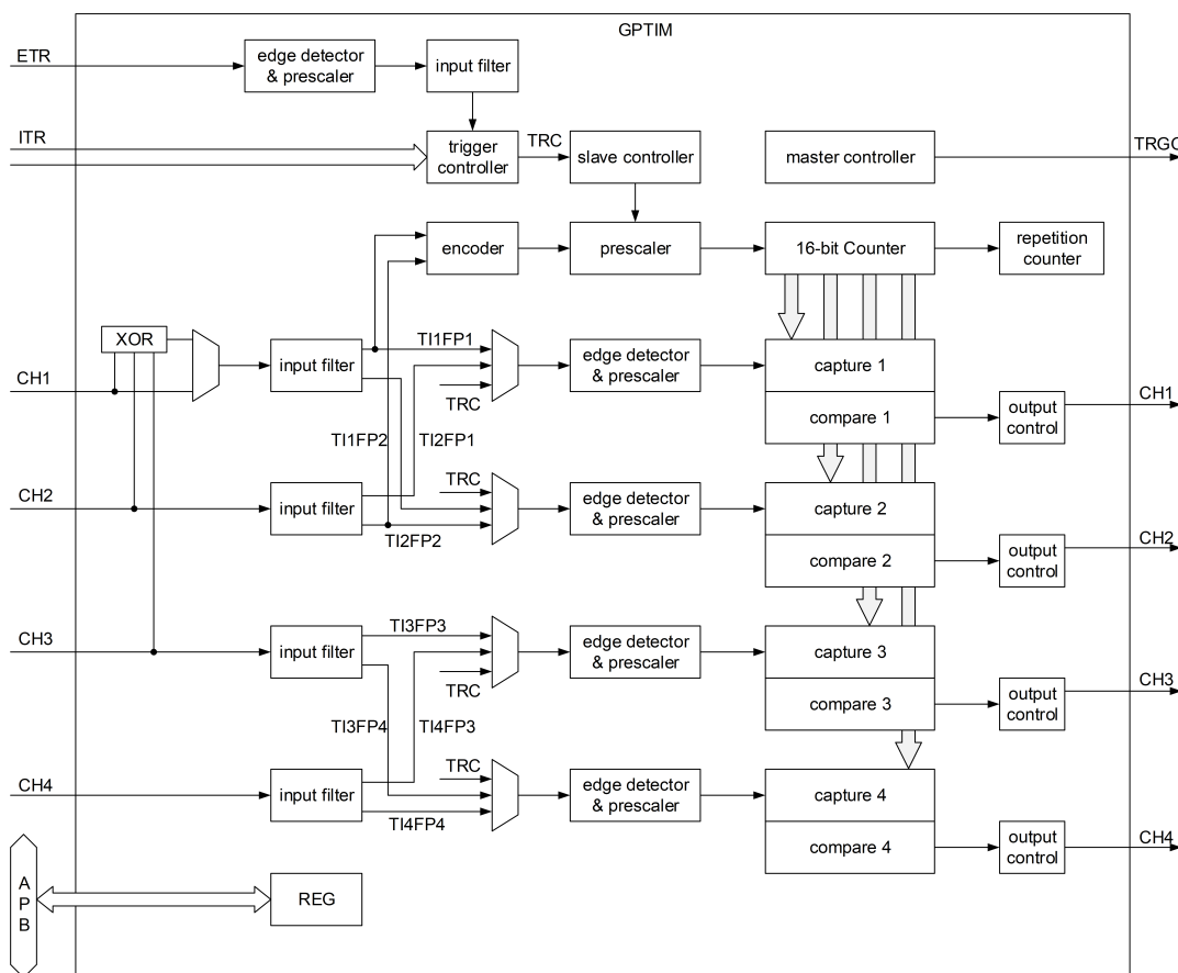
图 9-8: GPTIM 结构图
