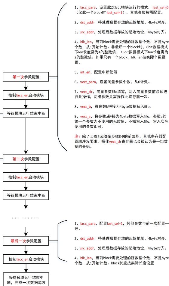
图 12-1: 非缓存模式下的配置流程图
