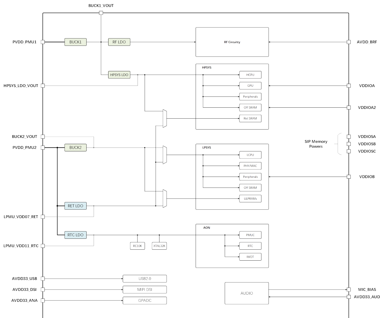
图 3-1: 电源管理架构
