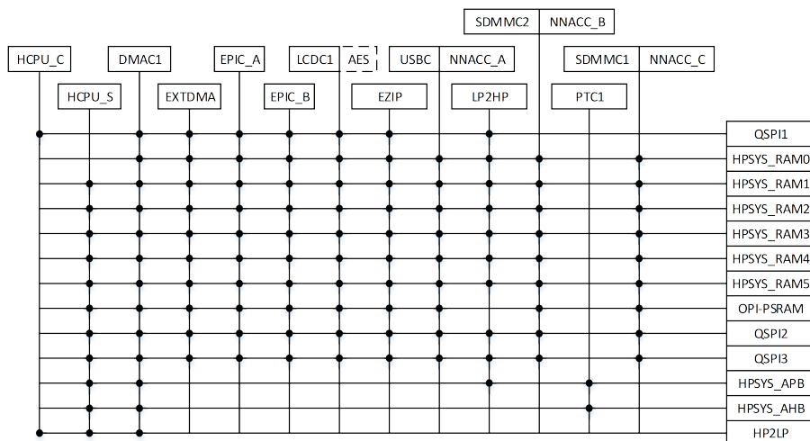
图 1-1: 性能处理器（大核）系统总线架构 HCPU
