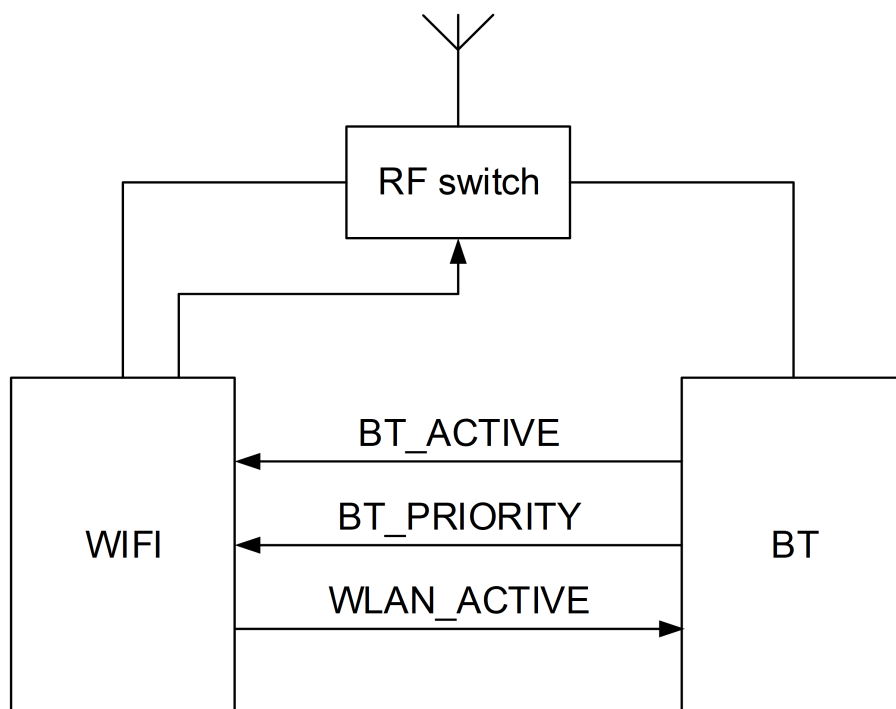
图 15-4: 外部仲裁的 3 线方案示例
