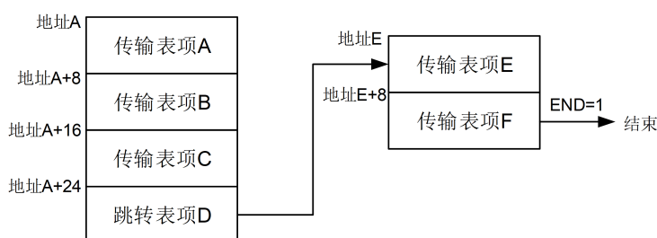
图 14-2: ADMA 链式描述表示例
