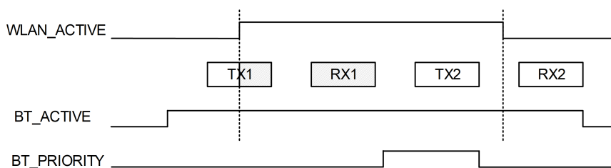
图 15-3: WLAN_ACTIVE 影响示例
