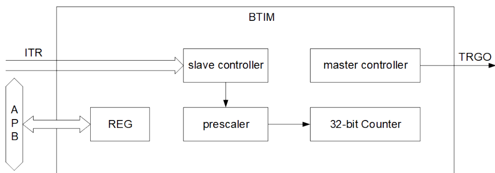
图 9-7: BTIM 结构图
