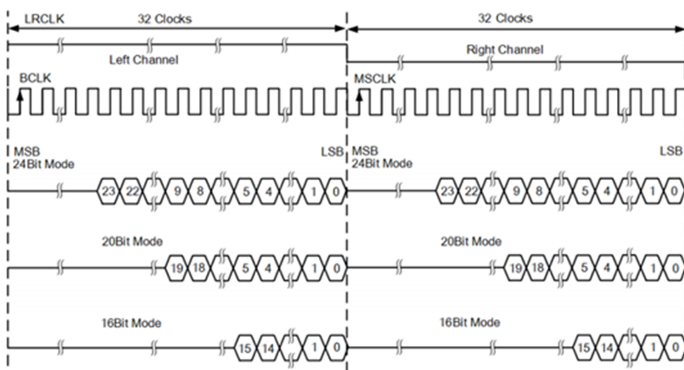
图 11-6: I2S 右对齐
