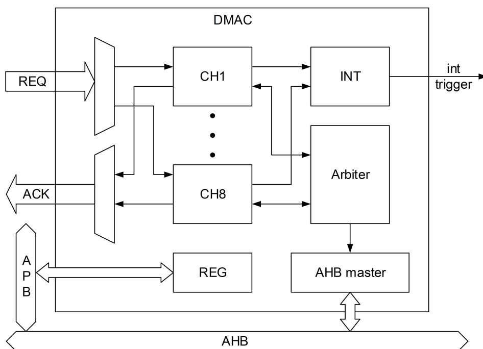
图 6-1: DMAC 结构图
