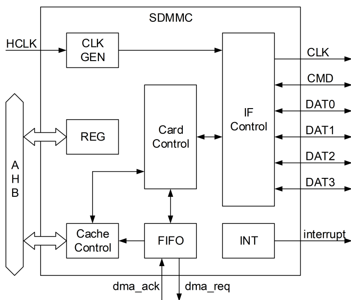
图 14-3: SDMMC 结构图
