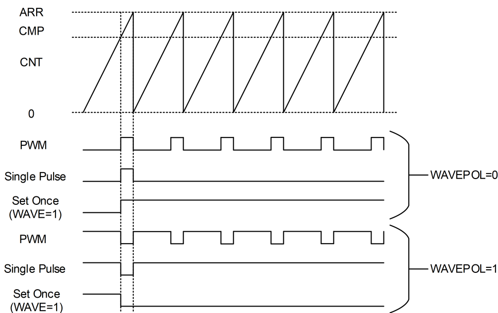
图 9-14: PWM 输出
