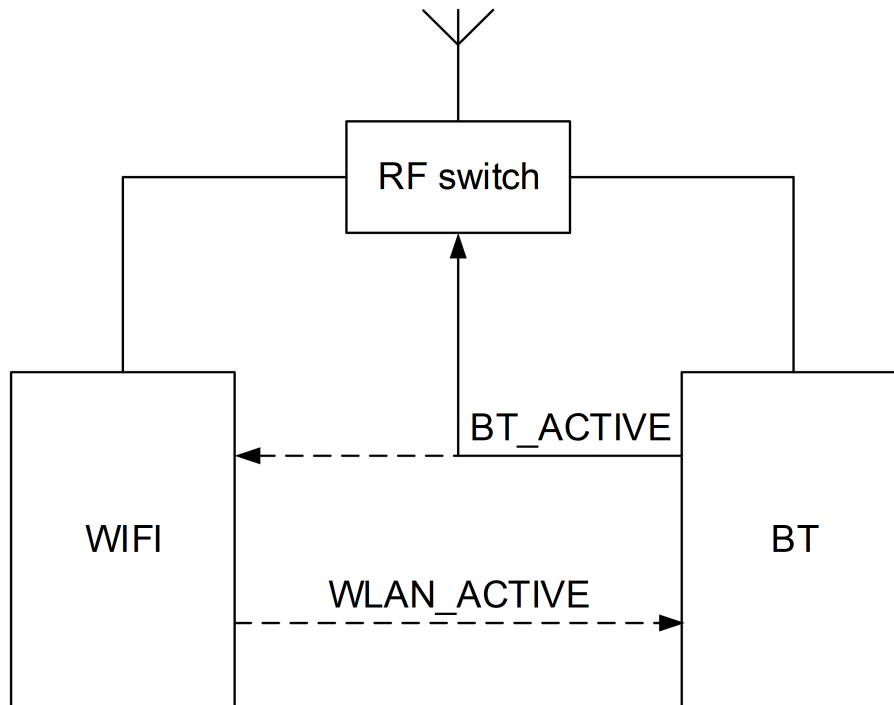
图 15-5: 内部仲裁的单线或 2 线方案示例
