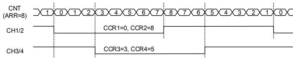
图 9-11: 不对称 PWM 输出
