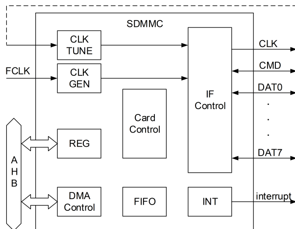
图 14-1: SDMMC 结构图
