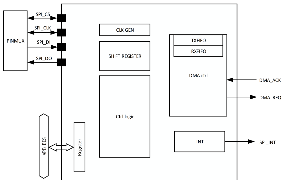
图 7-2: SPI 结构图
