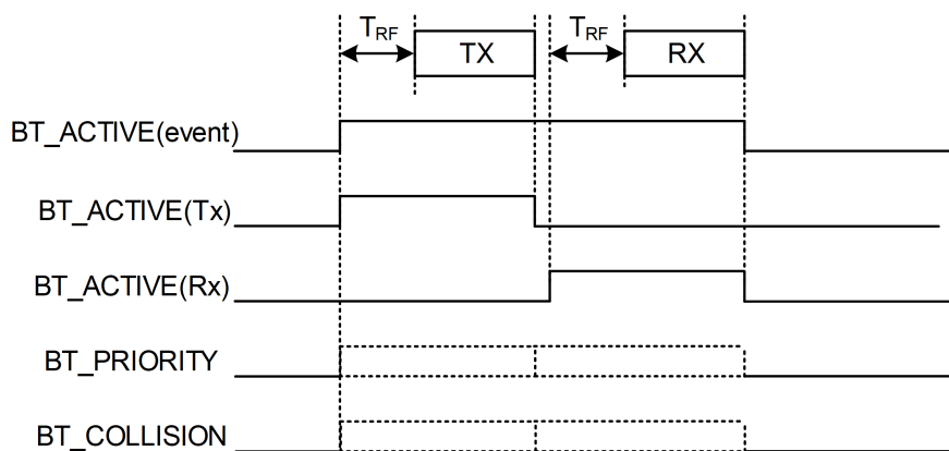
图 15-2: 输出信号示意图
