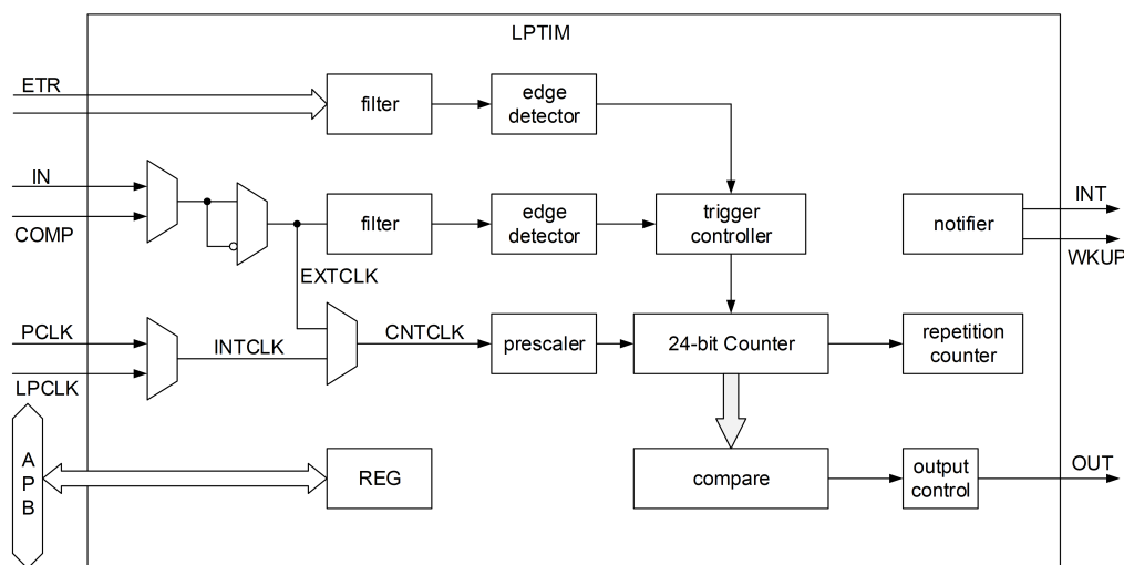
图 9-13: LPTIM 结构图
