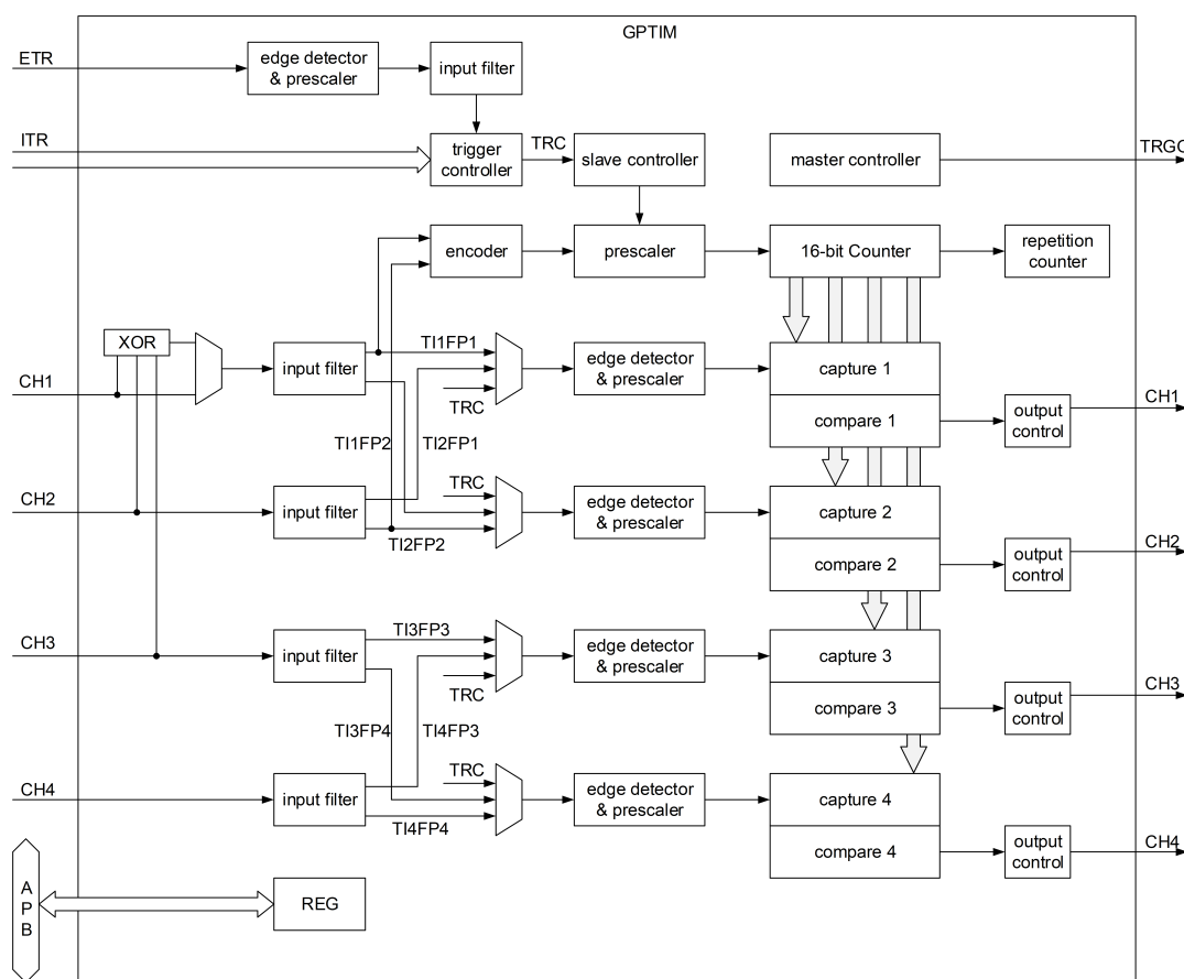
图 9-8: GPTIM 结构图
