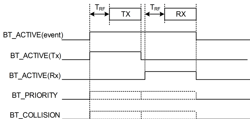
Figure 15-2: 输出信号示意图
