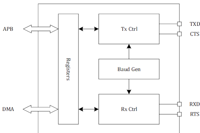
Figure 7-10: 通用异步收发器
