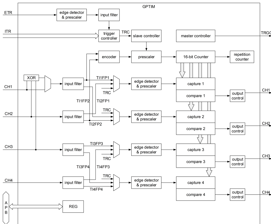
Figure 9-8: GPTIM 结构图
