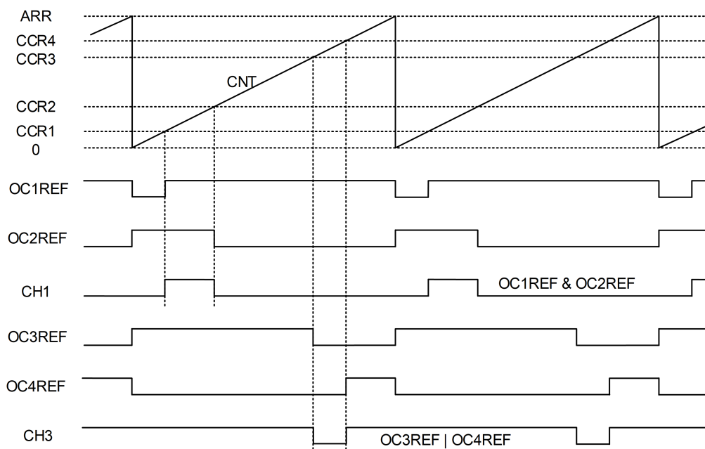
Figure 9-12: 组合 PWM 输出
