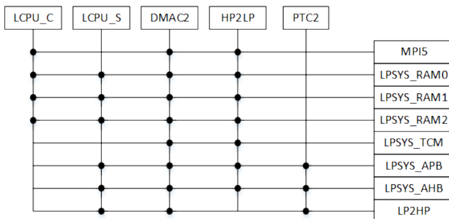
Figure 1-2: 低功耗处理器（小核）系统总线架构
