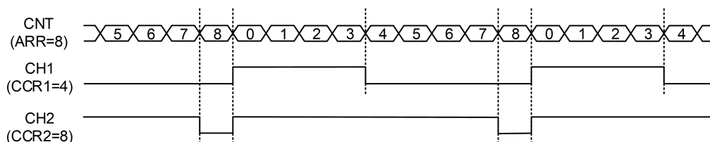
Figure 9-2: 递增计数模式下的 PWM 输出
