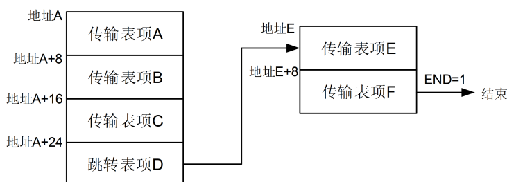
Figure 14-2: ADMA 链式描述表示例
