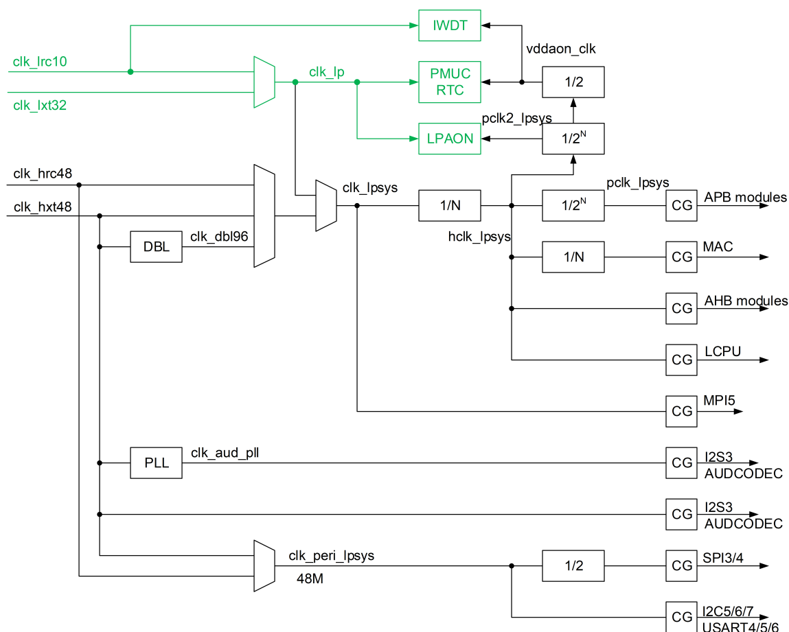
Figure 2-2: LPSYS 时钟结构
