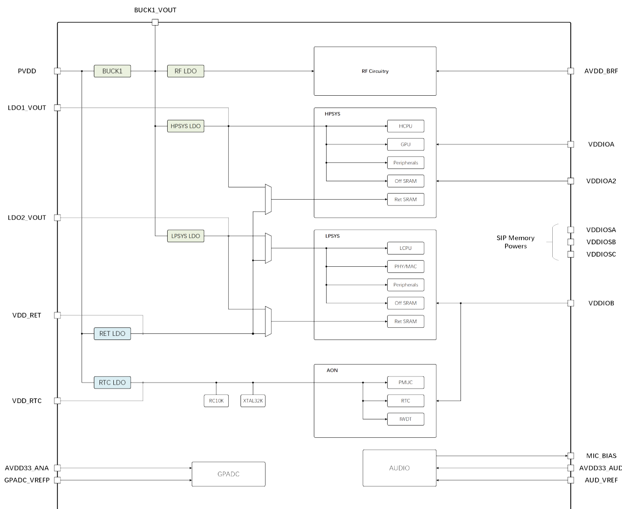
Figure 3-1: BGA 封装电源管理架构
