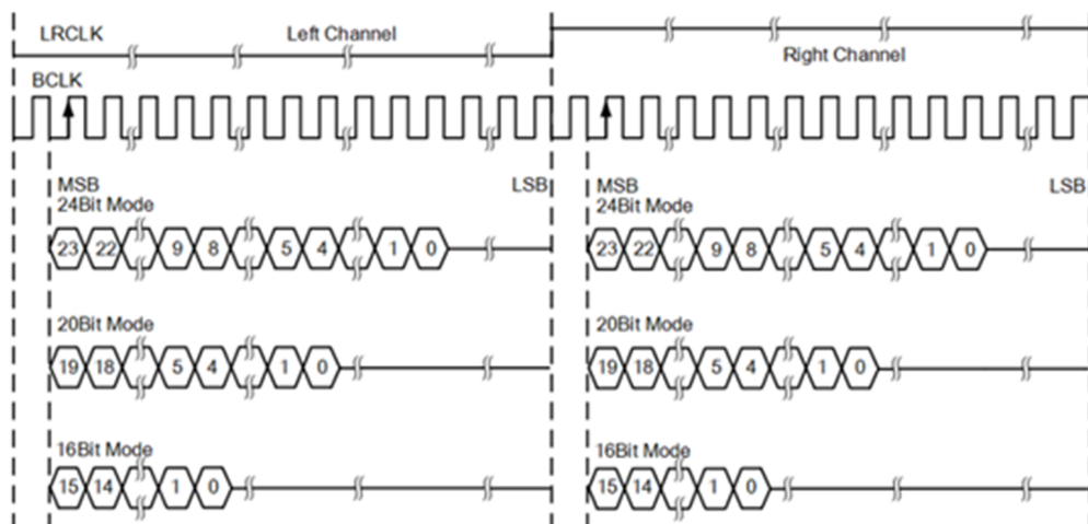
Figure 11-4: I2S 标准模式
