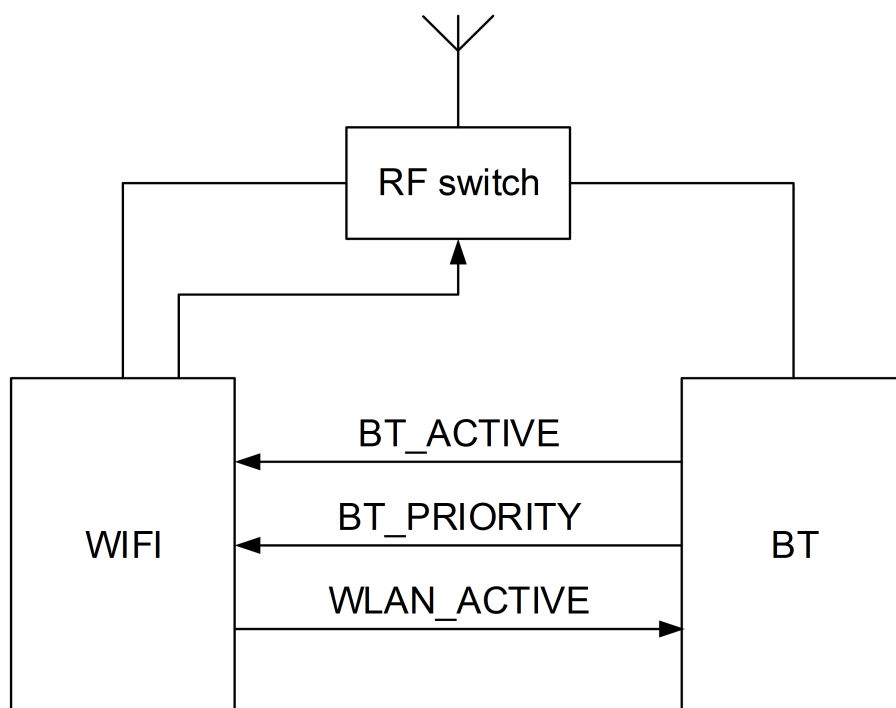
Figure 15-4: 外部仲裁的 3 线方案示例
