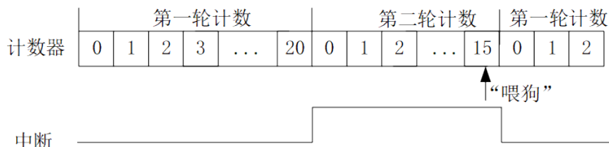
Figure 9-18: 模式 2 在第二轮计数时“喂狗”操作对计数器的影响, 第一轮计数时的影响和模式 1 相同 (假定超时值为 20)
