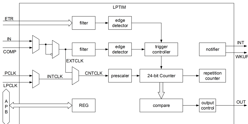
Figure 9-13: LPTIM 结构图
