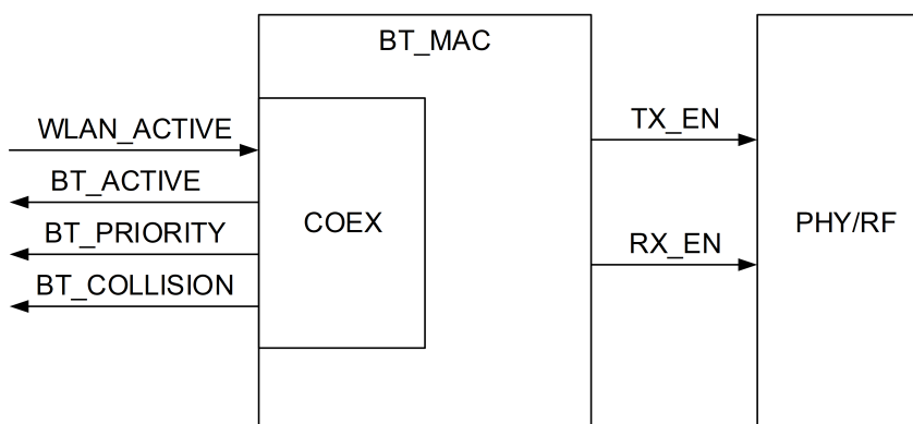
Figure 15-1: 蓝牙共存示意图
