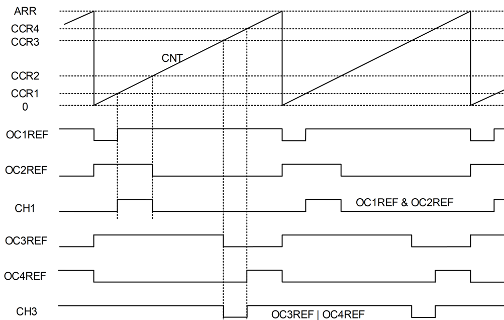
Figure 9-5: 组合 PWM 输出
