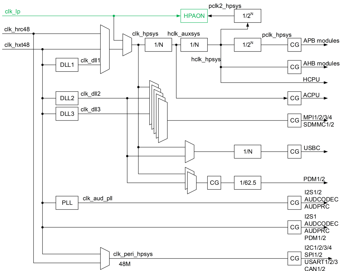
Figure 2-1: HPSYS 时钟结构
