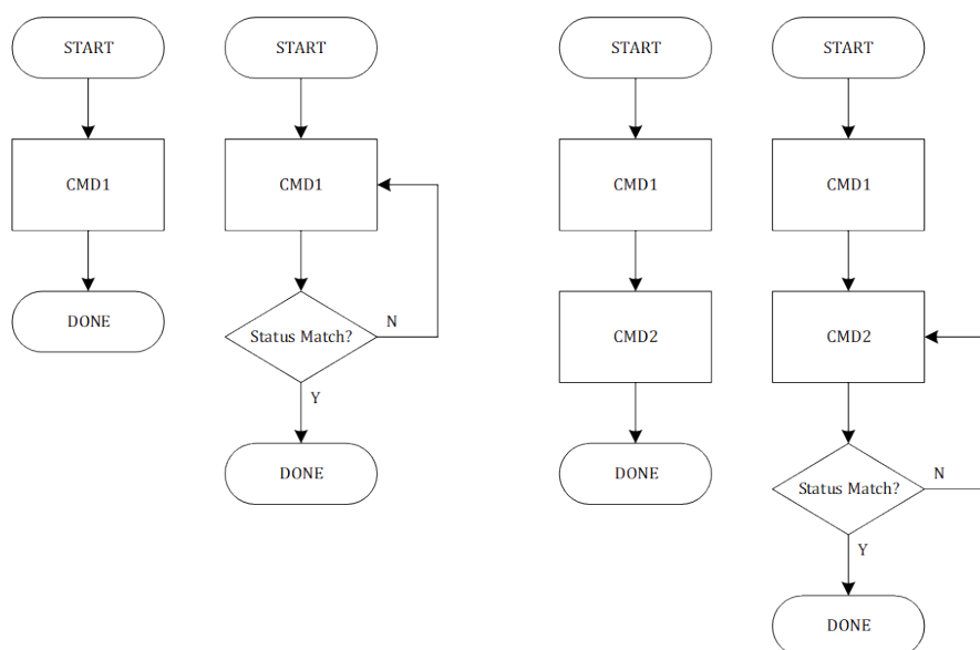
Figure 14-5: 寄存器模式单个和多个命令时序的序列
