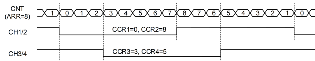
Figure 9-11: 不对称 PWM 输出
