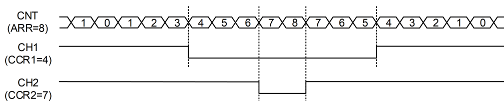
Figure 9-3: 中心对齐计数模式下的 PWM 输出
