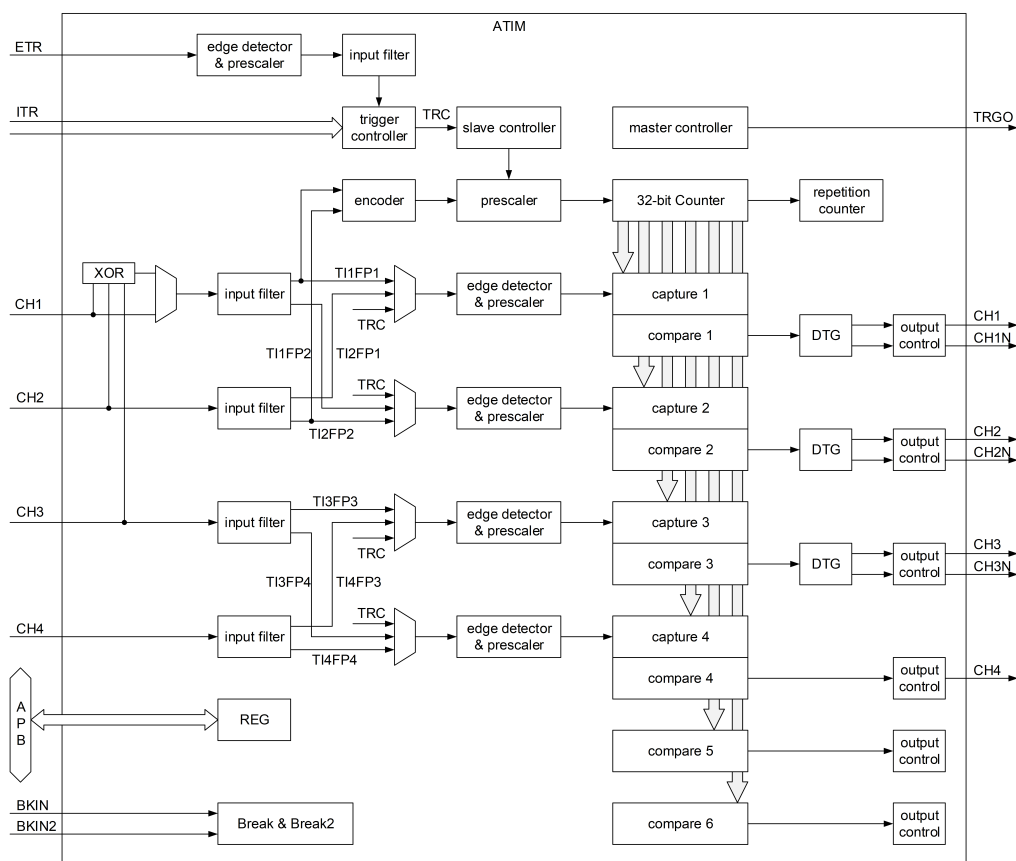
Figure 9-1: ATIM 结构图
