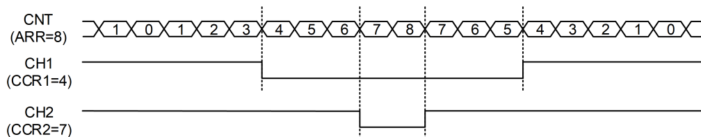
Figure 9-10: 中心对齐计数模式下的 PWM 输出
