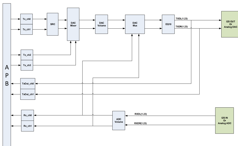
Figure 11-7: Audprc 结构图
