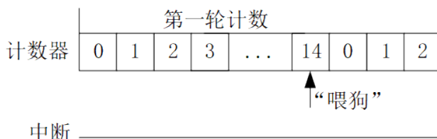
Figure 9-17: 模式 1 “喂狗”行为对计数器的影响 (假定超时值为 20)
