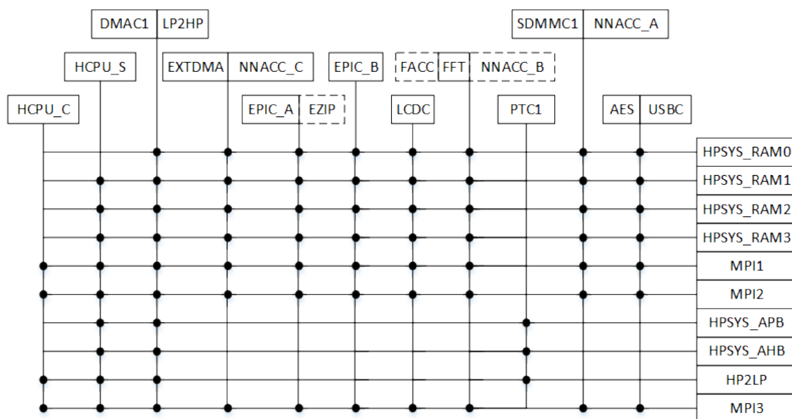
Figure 1-1: 性能处理器（大核）系统总线架构
