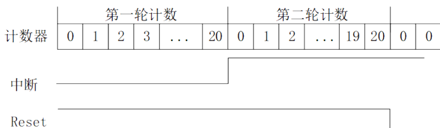
Figure 9-16: 模式 2 的中断以及 reset 信号产生与计数器的关系 (假定超时值为 20, reset 低有效)
