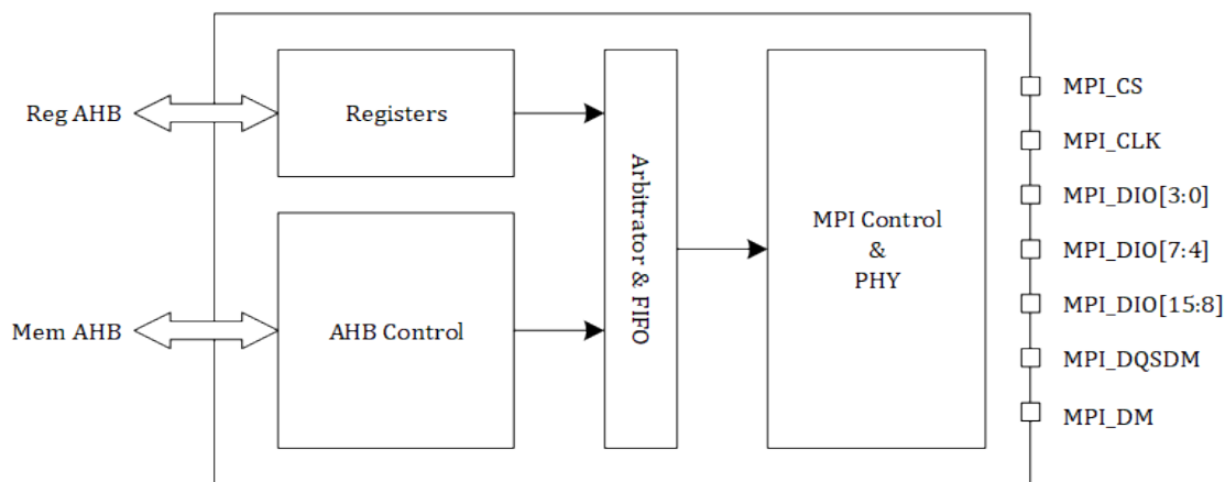
Figure 14-4: MPI 控制器框图
