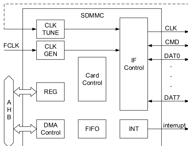
Figure 14-1: SDMMC 结构图
