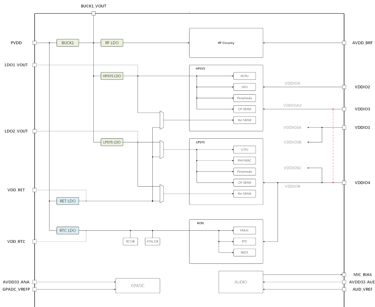
Figure 3-2: QFN 封装电源管理架构
