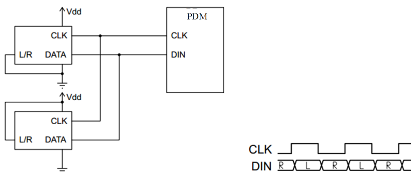
Figure 11-1: 数字麦克风通过 PDM 模块的典型连接
