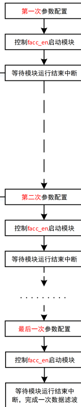
Figure 12-2: 缓存模式下的配置流程图
