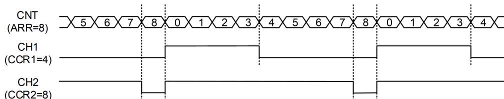
Figure 9-9: 递增计数模式下的 PWM 输出
