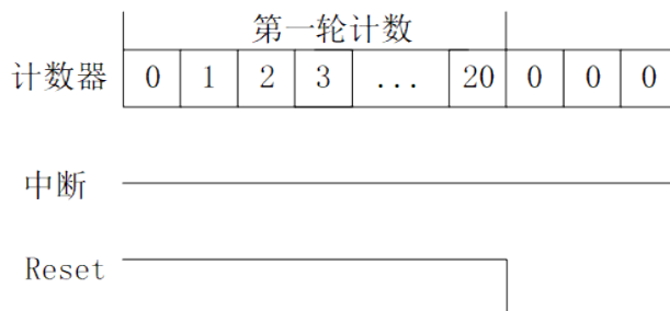
Figure 9-15: 模式 1 的中断以及 reset 信号产生与计数器的关系 (假定超时值为 20, reset 低有效)
