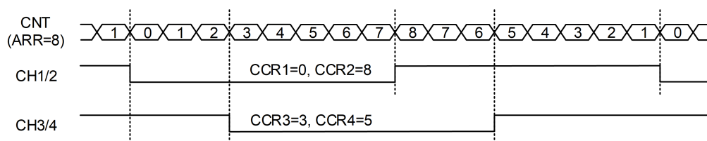
Figure 9-4: 不对称 PWM 输出
