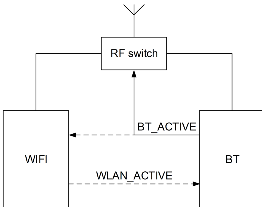
Figure 15-5: 内部仲裁的单线或 2 线方案示例
