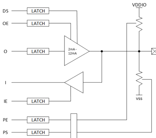
Figure 5-1: IO 结构
