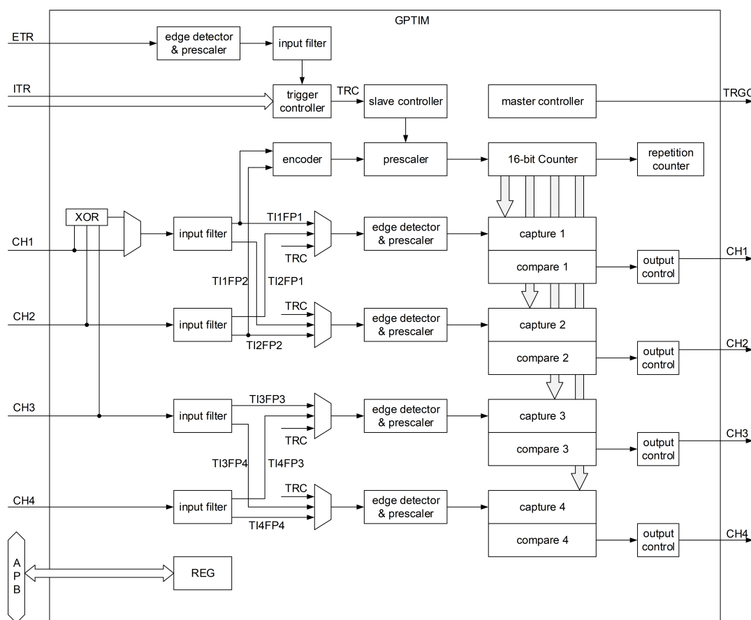
图 9-2: GPTIM 结构图
