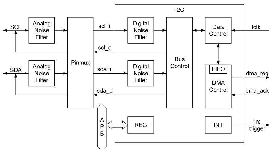
图 7-1: I2C 结构图
