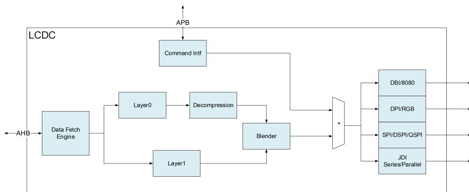
图 10-1: LCDC 架构图
