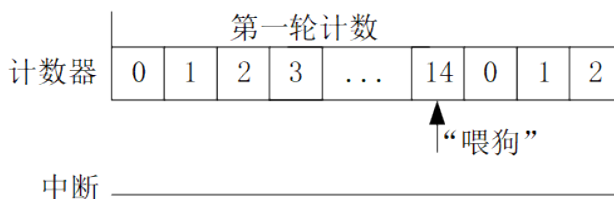
图 9-11: 模式 1 “喂狗”行为对计数器的影响（假定超时值为 20）
