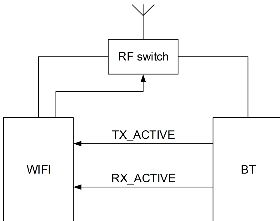
图 15-2: 外部仲裁的 2 线方案示例
