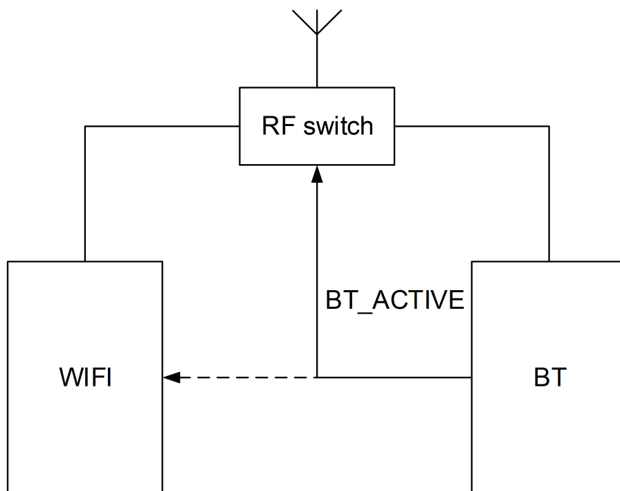
图 15-3: 内部仲裁的单线方案示例
