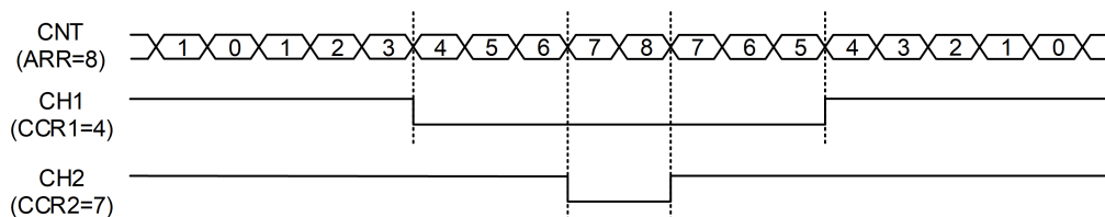
图 9-4: 中心对齐计数模式下的 PWM 输出
