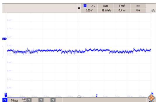
图 3-22: LDO 负载响应, I_{OUT, LDO} : 10uA-1mA
