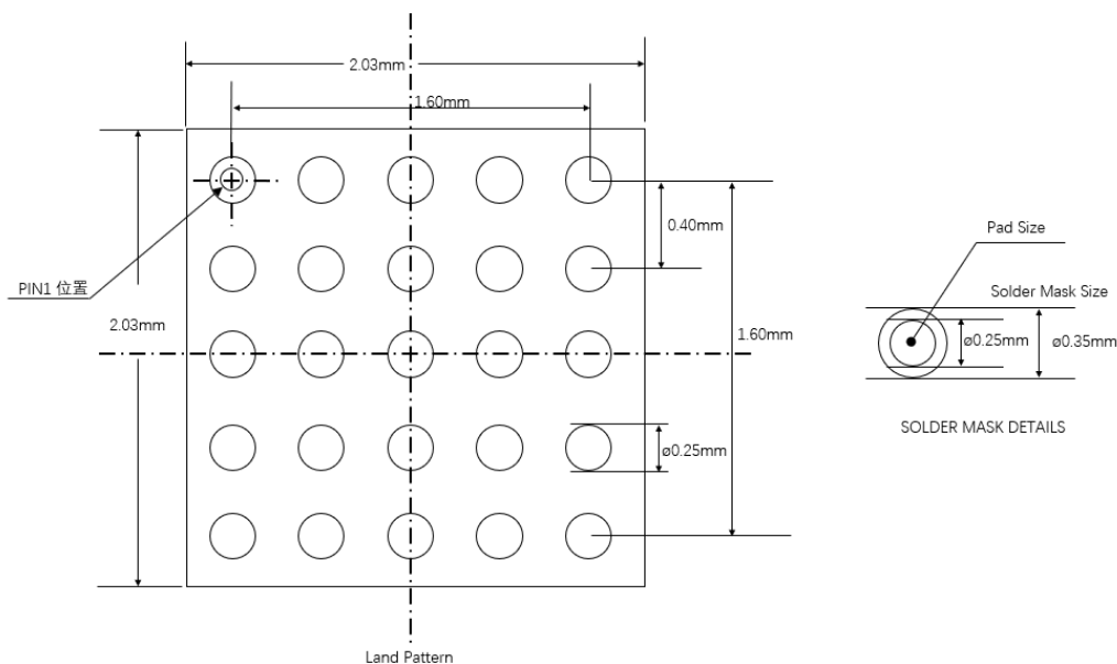
图 6-2: 焊盘尺寸
