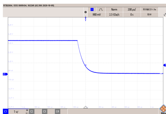
图 3-28: HVSW 关断时间, HVSW 空载
