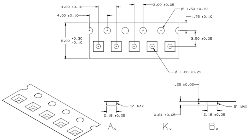
图 6-4: 卷带尺寸
