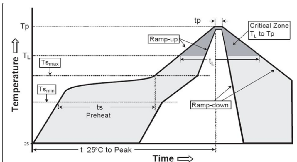
图 6-5: 分级回流焊
