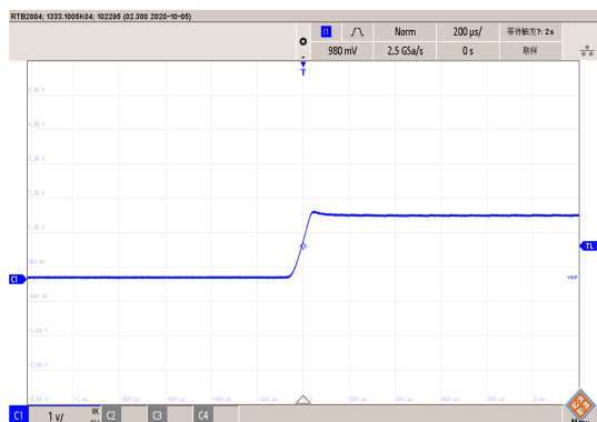
图 3-31: LVSW 上电时间, LVSW 空载
