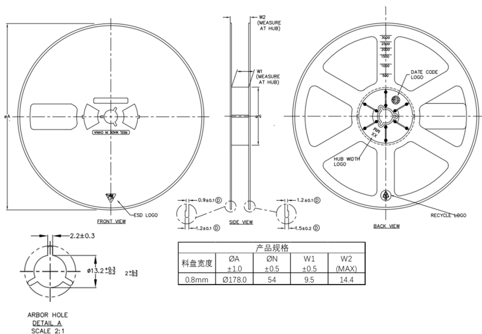
图 6-3: 料盘尺寸
