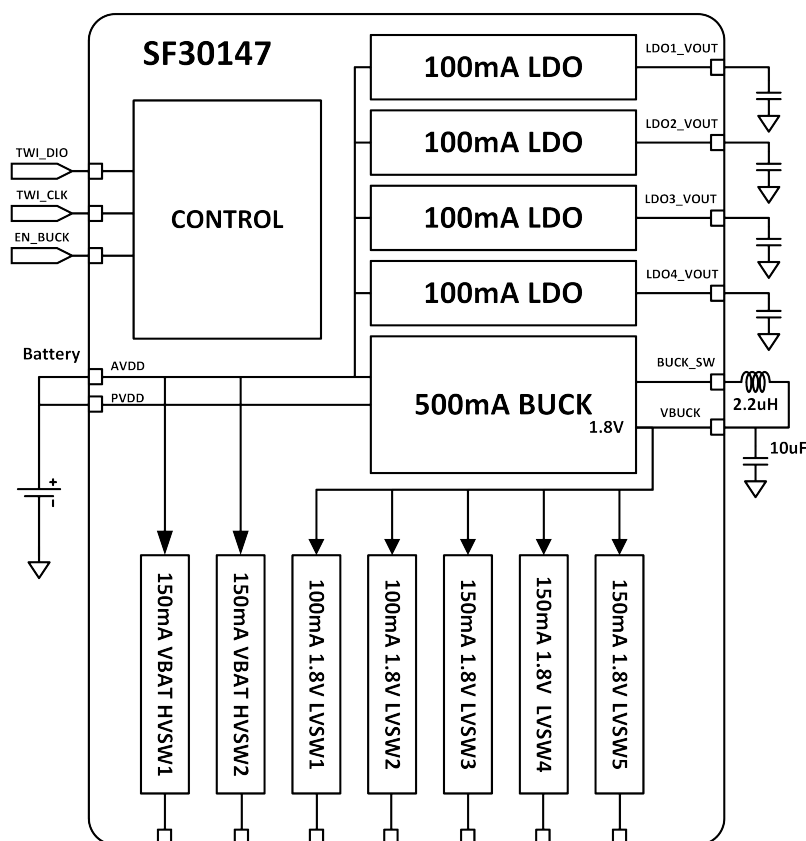
图 0-1: 功能框图
