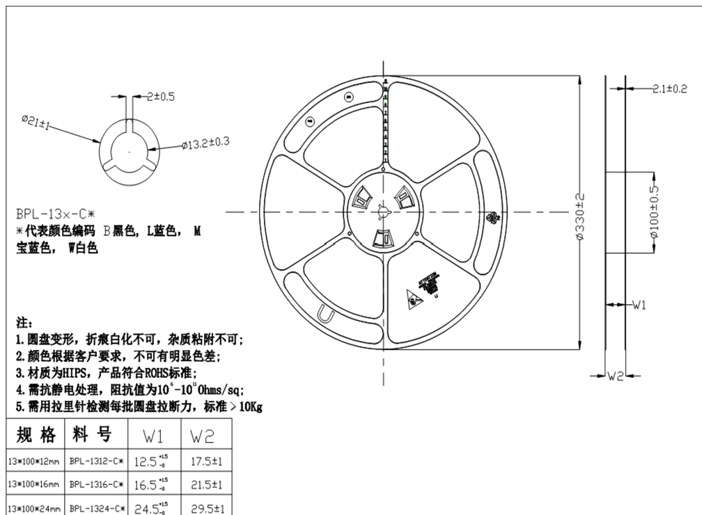
图 5-4: 卷盘尺寸
