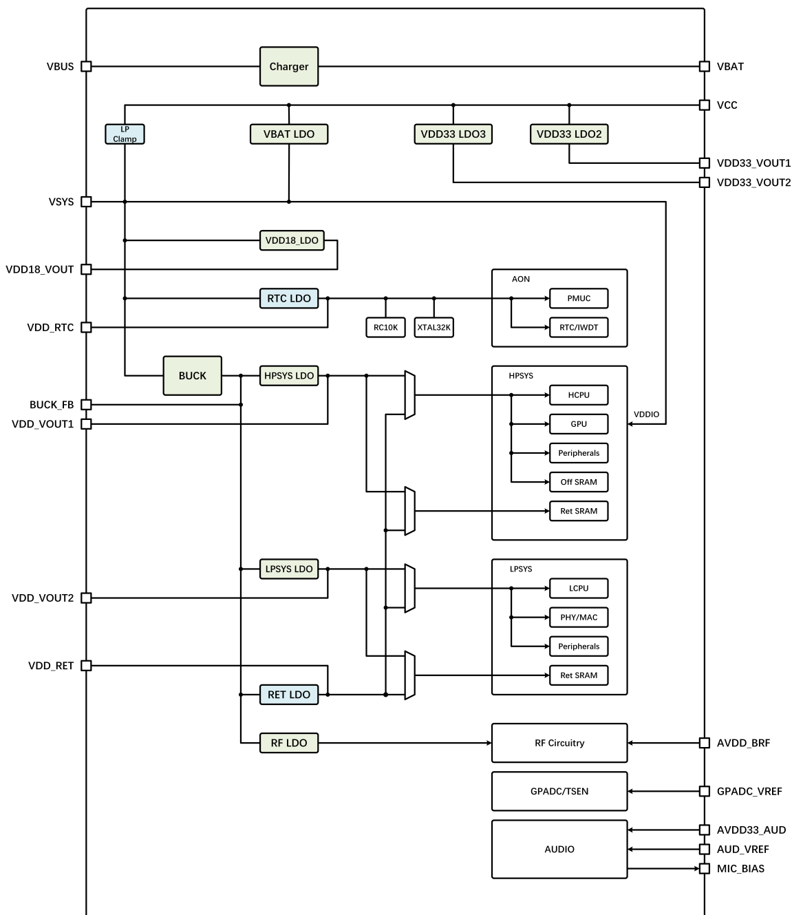
图 1-3: QFN 封装电源管理架构
