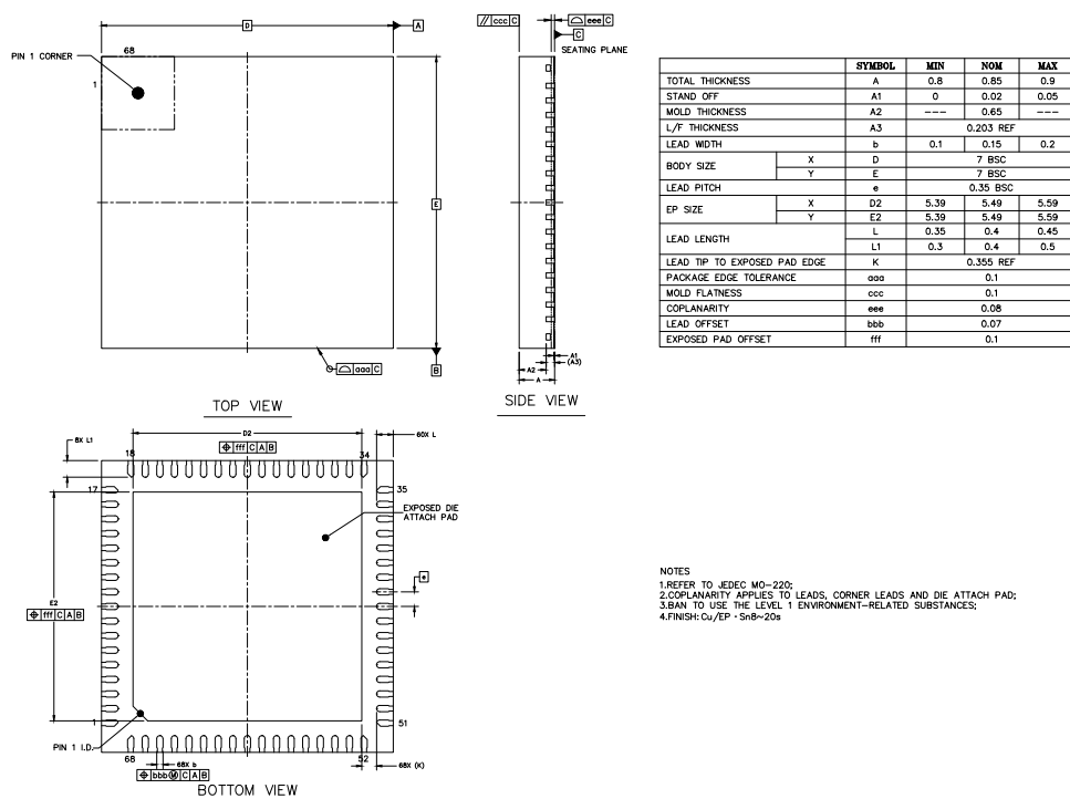
图 5-2: QFN68L 封装尺寸
