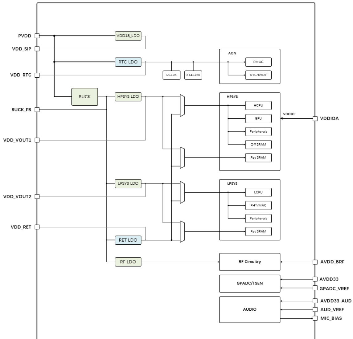
图 1-3: QFN 封装电源管理架构
