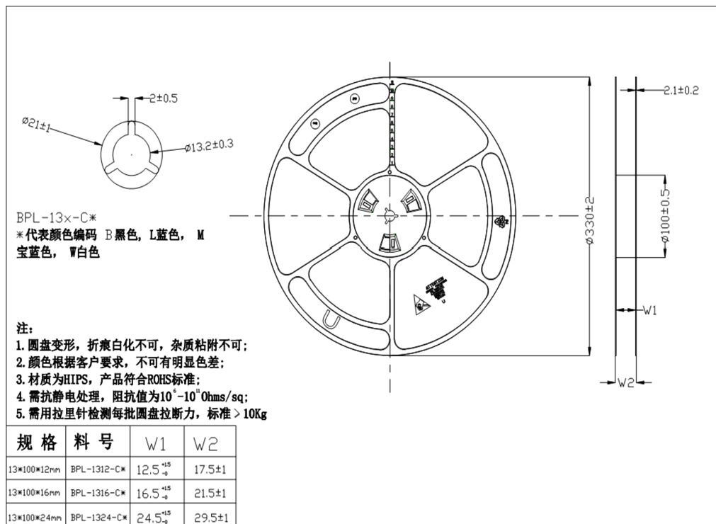
图 5-4: 卷盘尺寸
